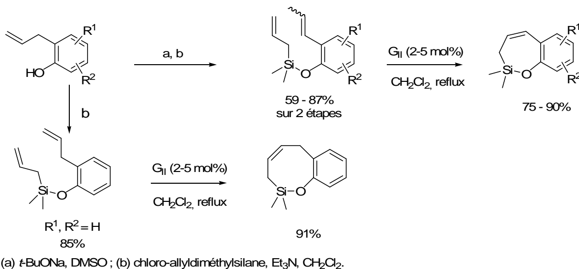
Schéma II-24 : Formation d'aryles siloxanes
