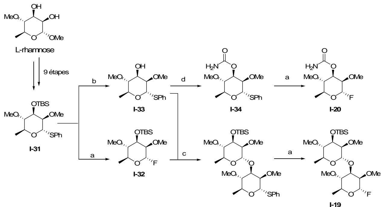
Schéma I-4 : Synthèse des fluoro-sucres
