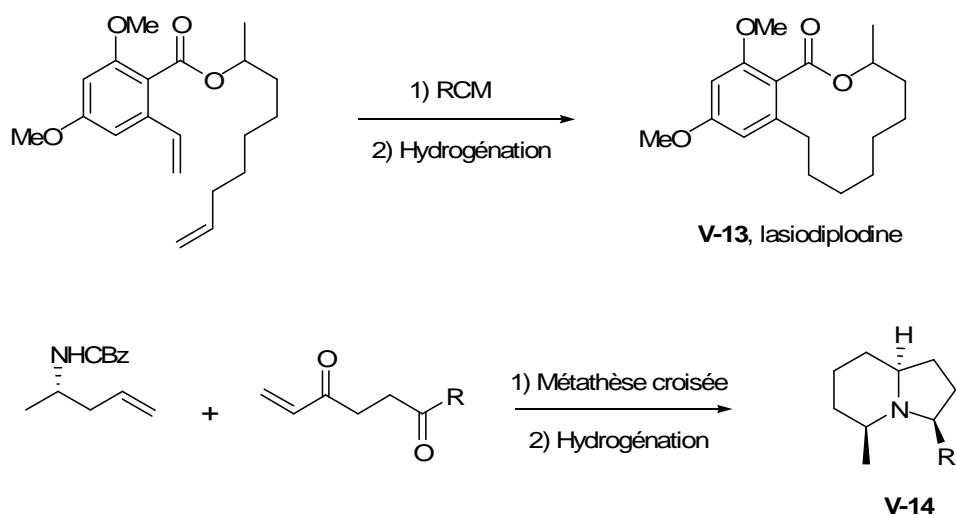
Schéma V-7 : Processus séquentiel métathèse / hydrogénation
