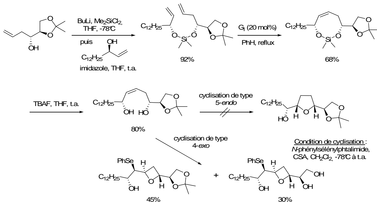
Schéma II-37 : Formation d'oxétane par séleoétherification
