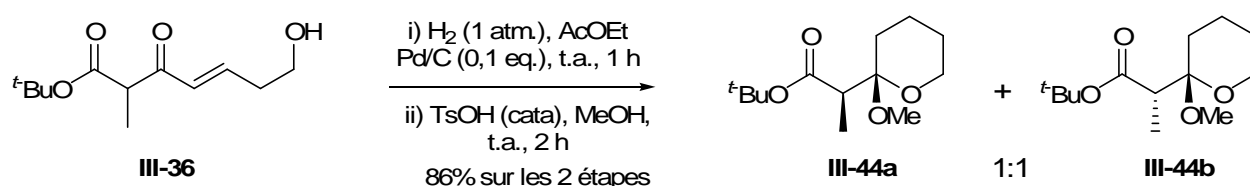
Schéma III-11
