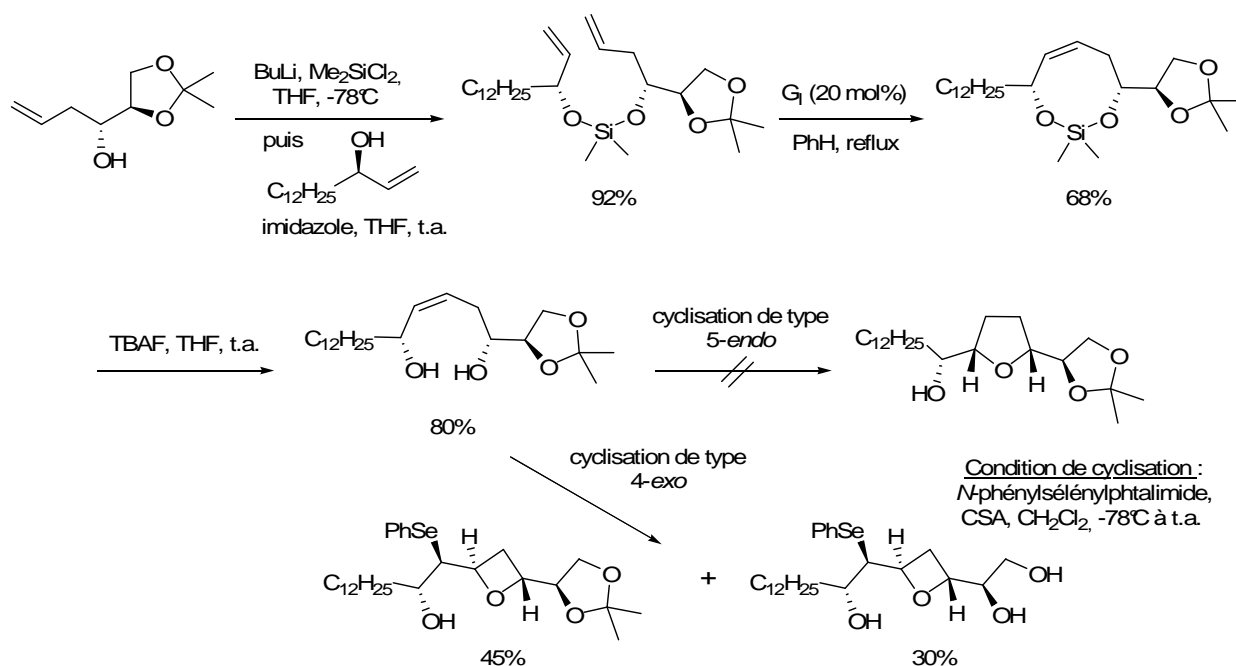
Schéma II-37 : Formation d'oxétane par sélénoétherification
