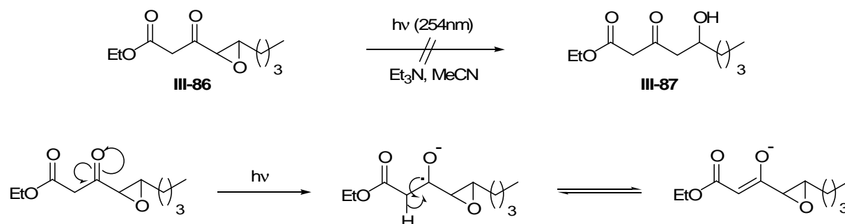
Schéma III-29 : Tentative d'ouverture régiosélective par voie photochimique
