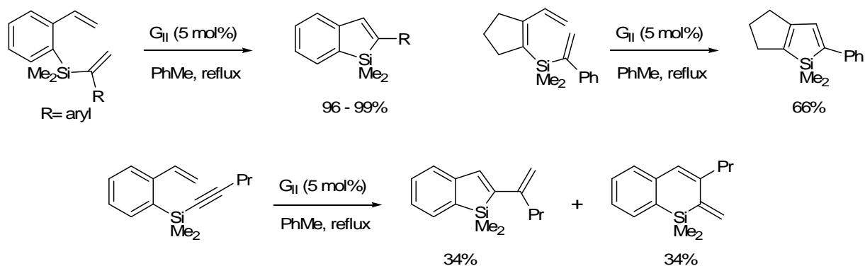
Schéma II-54 : Formation de composés de type silacyclopentadiènes
