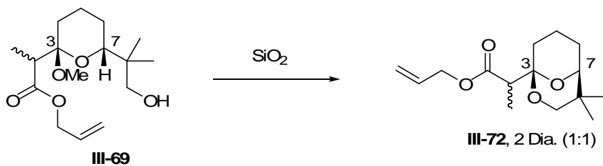
Schéma III-20 : Formation du composé bicyclique III-72
