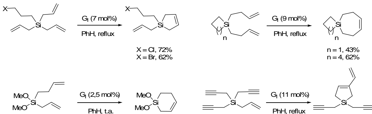
Schéma II- 52 : Formation de silacycloalcènes
