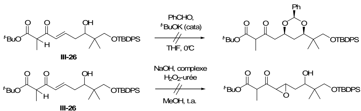
Schéma III-25 : Tentatives d'addition de type-1,4 sur le composé ( III-26 )
