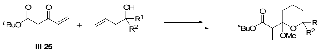
Schéma III-10 : Stratégie d'obtention des analogues
