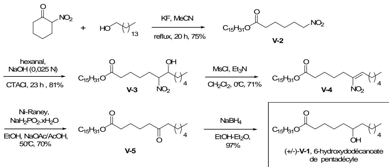
Schéma V-1 : Synthèse du 6-hydroxydodécanoate de pentadécyle selon Ballini
