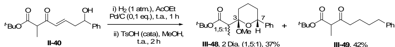
Schéma III-12
