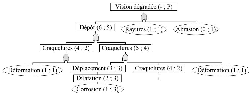
Figure 43 : Extrait d'un arbre des défaillances d'une fenêtre
