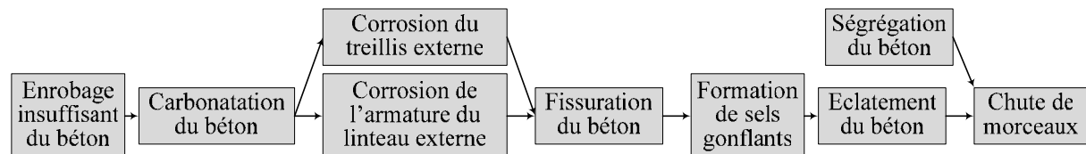
Figure 75 : Scénario de « chute de morceaux » du mur en béton
