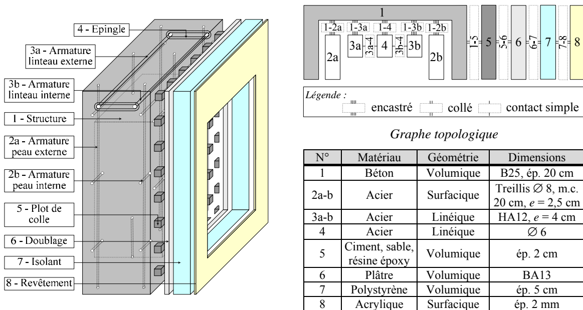
Grphe structurel éclaté en 3D
