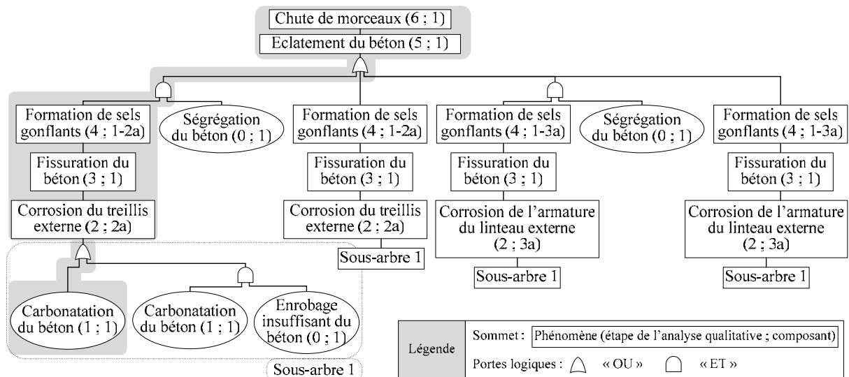
Figure 76 : Arbre des défaillances du scénario de « chute de morceaux » du mur en béton
