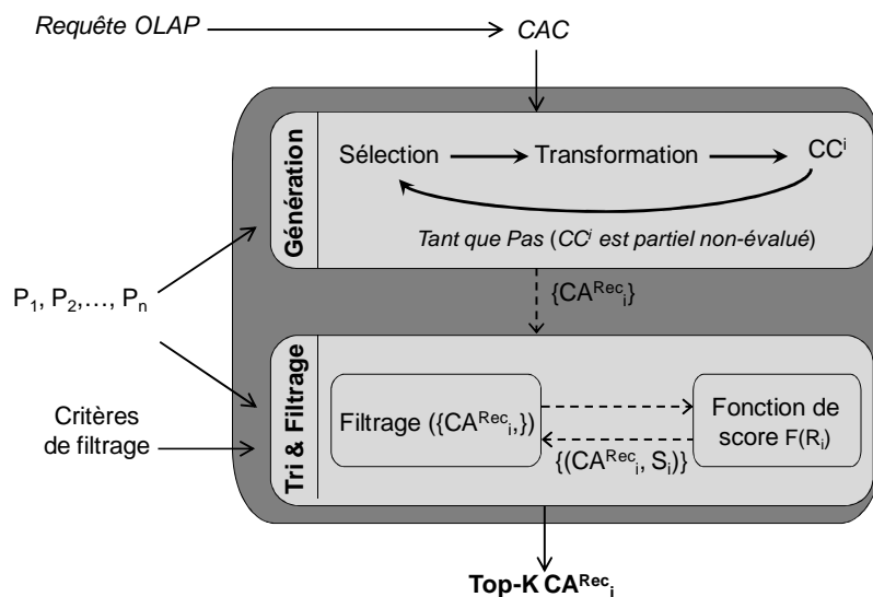
Figure 32. Mécanisme de construction des recommandations OLAP
