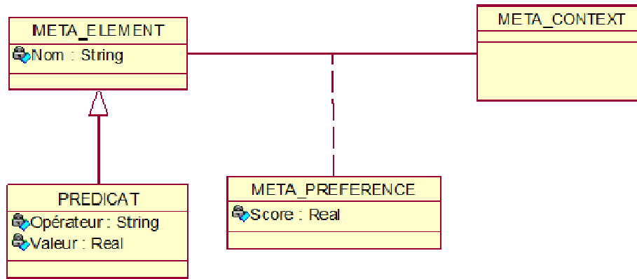
Figure 17. Modèle d'un profil utilisateur (représenté au format UML)
