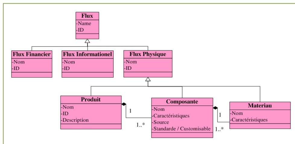
Figure 31 : diagramme de classes des Flux
