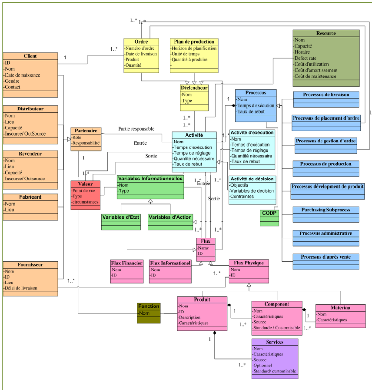
Figure 33 : Diagramme de classe des éléments de notre modèle conceptuel
