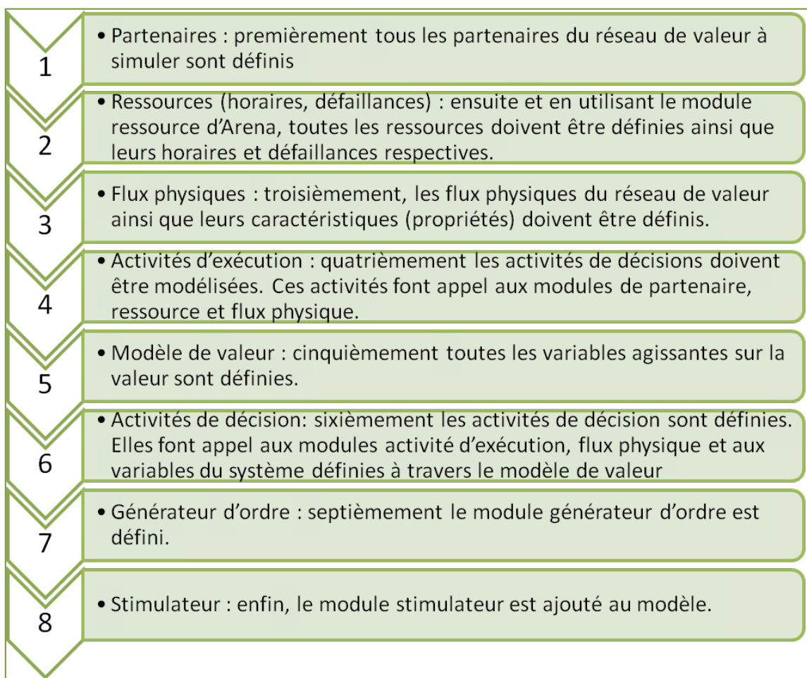
Figure 58 : Ordre de placement des modules pour construction du modèle de simulation
