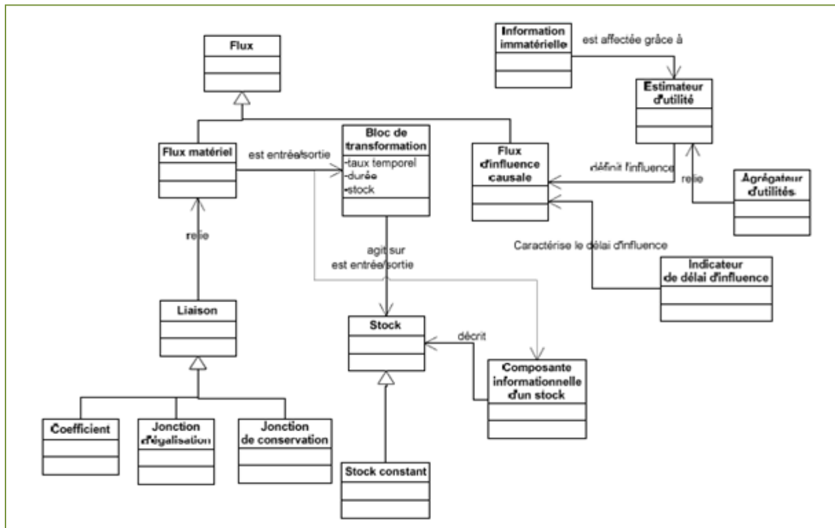
Figure 16 : Diagramme de classes UML des éléments de modélisation SimulValor (Mauchand, 2007).
