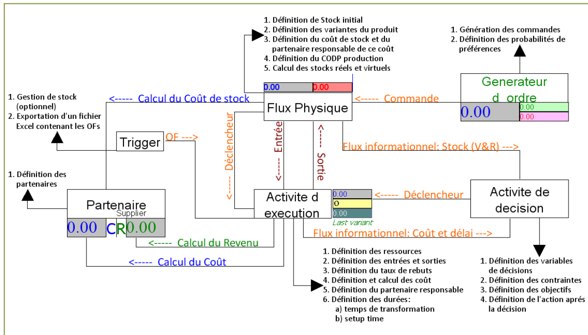
Figure 57 : Liens entre les principaux modules de notre librairie
