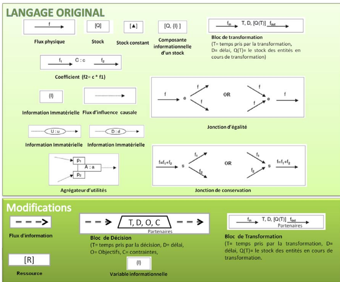
Figure 38 : Modifications proposées au langage SimulValor.
