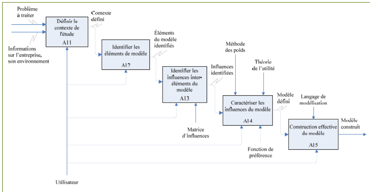
Figure 14. Construction du modèle SimulValor extrait de (Mauchand, 2007).
