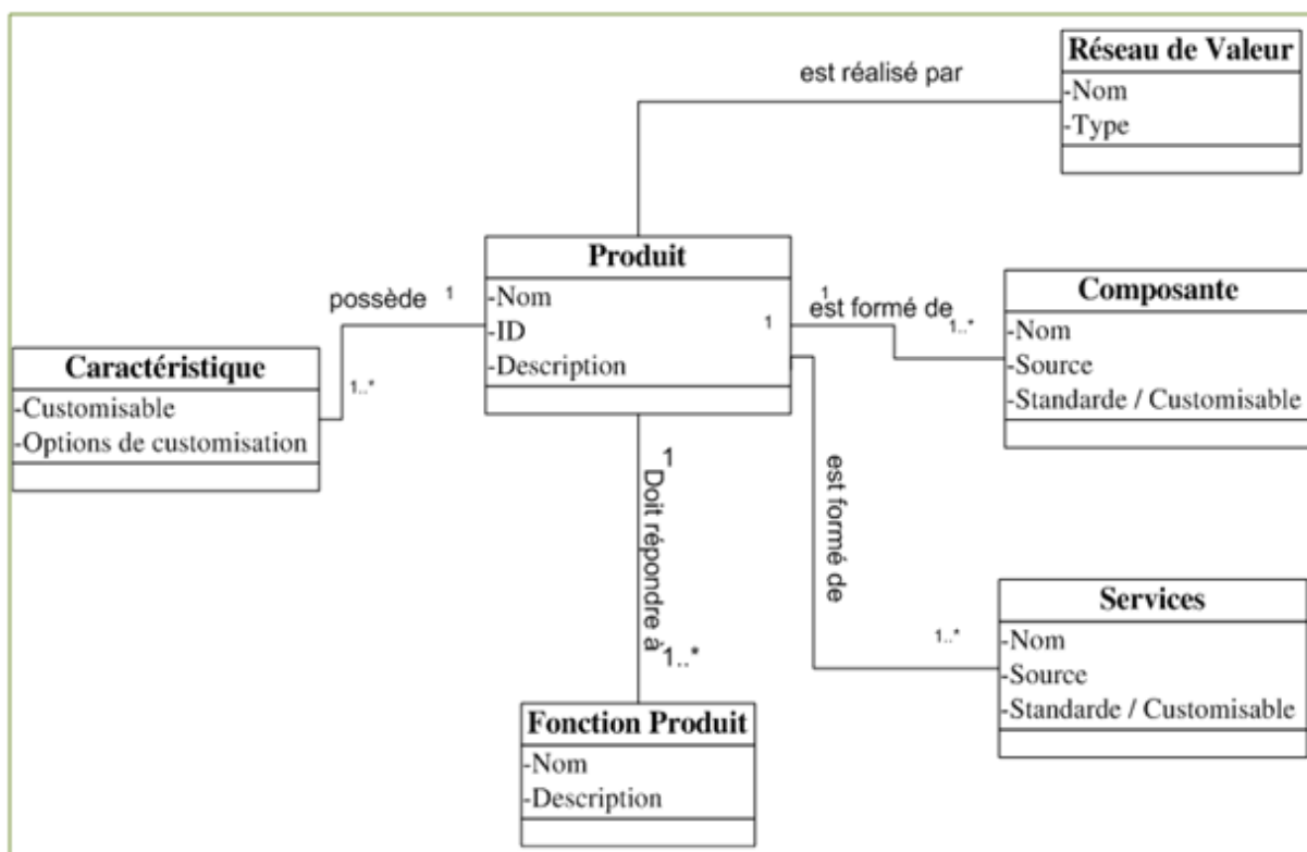
Figure 32 : Modèle objet : Produit
