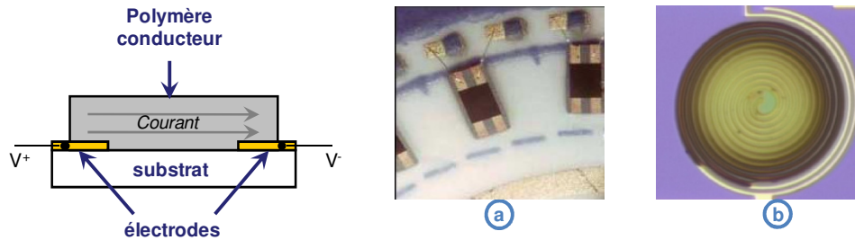
Figure I-3 : Schéma de principe d'un capteur à polymère conducteur et photographie de capteurs polymères conducteurs sur électrode simple (source ctib-tchn) (a) et sur électrodes interdigitées spirales (Li et al., 2007a) (b)
