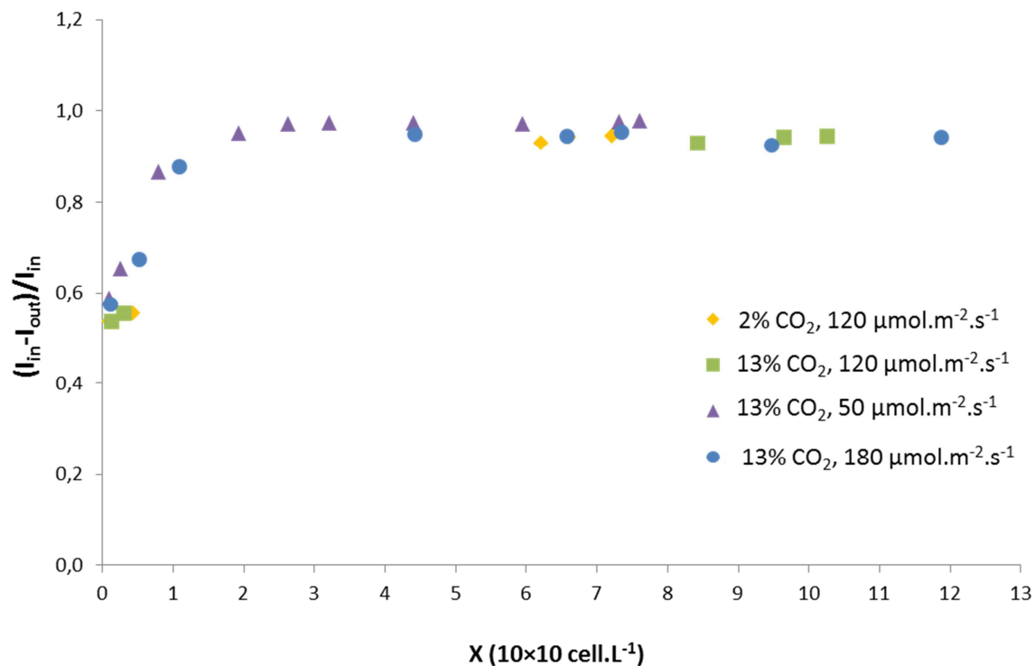
Figure III.8. Absorption de la lumière dans le réacteur en fonction de la concentration cellulaire de C. vulgaris lors des différentes cultures en batch (2% et 13% de CO 2 , 50 µmol.m -2 .s -1 , 120 µmol.m -2 .s -1 et 180 µmol.m -2 .s -1 )
