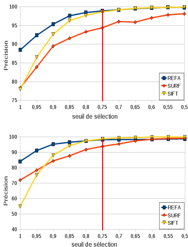
FIG. 3.12 – Détermination du seuil de sélection pour un changement de point de vue de 20^\circ (haut) et un couplage rotation/changement d'échelle de 40^\circ/1,35 (bas).
