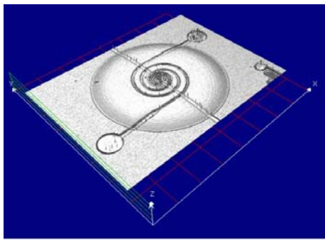
FIGURE 34 : A) IMAGE 3D DE LA PLATEFORME CHAUFFANTE FOURNIE PAR LE PROFILOMETRE INTERFEROMETRIQUE ; B) DEFORMATIONS DE LA PLATEFORME POUR DIFFERENTES TENSIONS APPLIQUEES SUR LE HEATER
