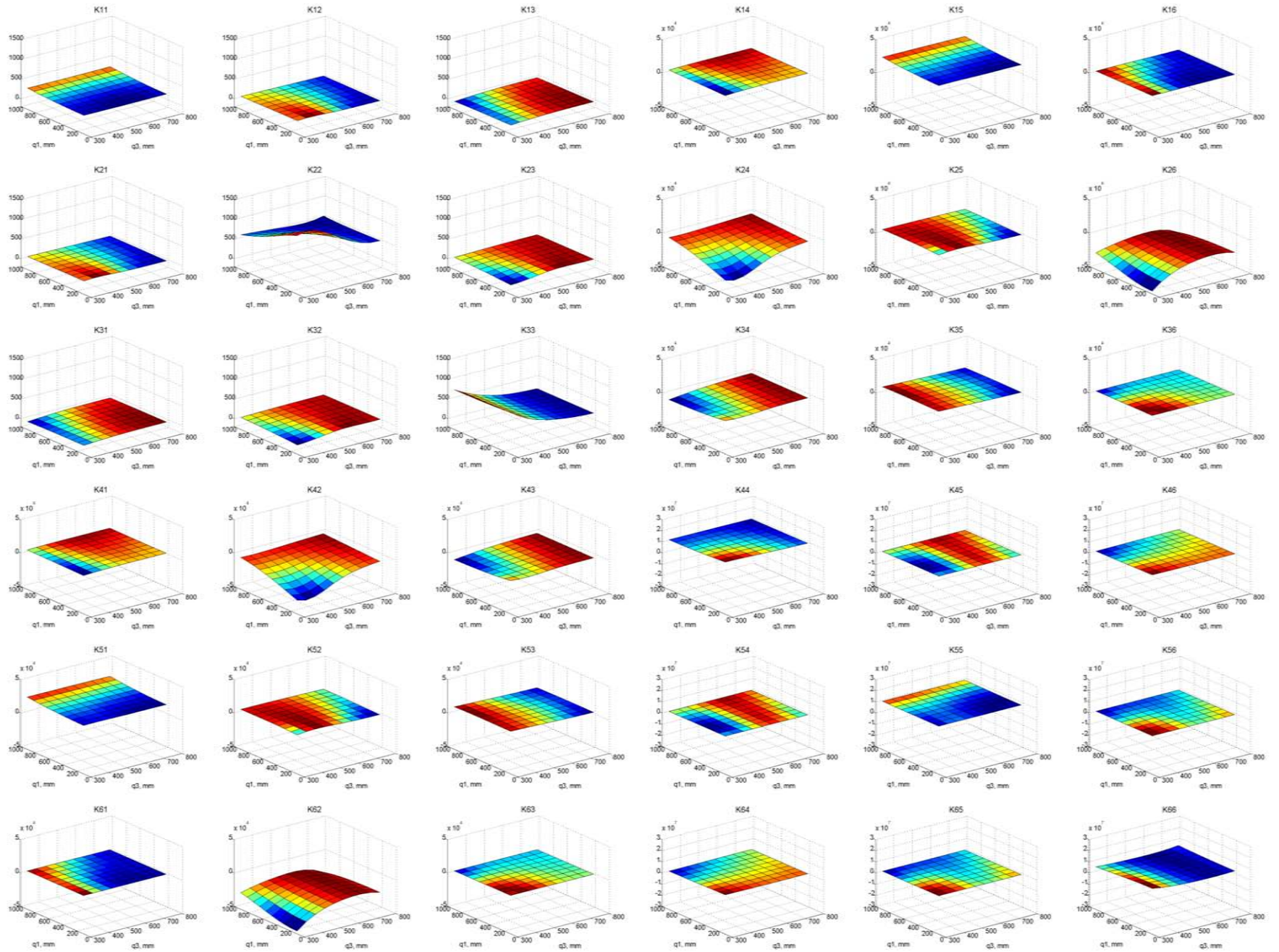
Cartes de rigidité de l'isoglide4-T3R1 condensée à son point caractéristique P pour q_2 = 250 \text{ mm} \varphi_P = 0^\circ
