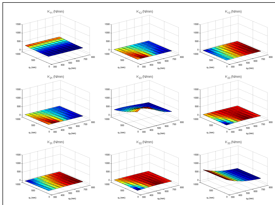
Figure 3-12 : Variations de K_{Fd} de l'ISOGLIDE3-T3 dans son espace de travail pour q_2=700\text{mm} (les grandeurs sont en \text{N/mm} ).
