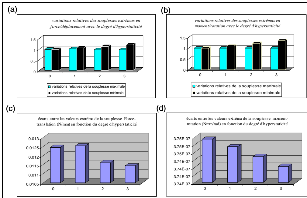
Figure 5-5 : Comparaison des souplesses extrémales des différentes versions.
