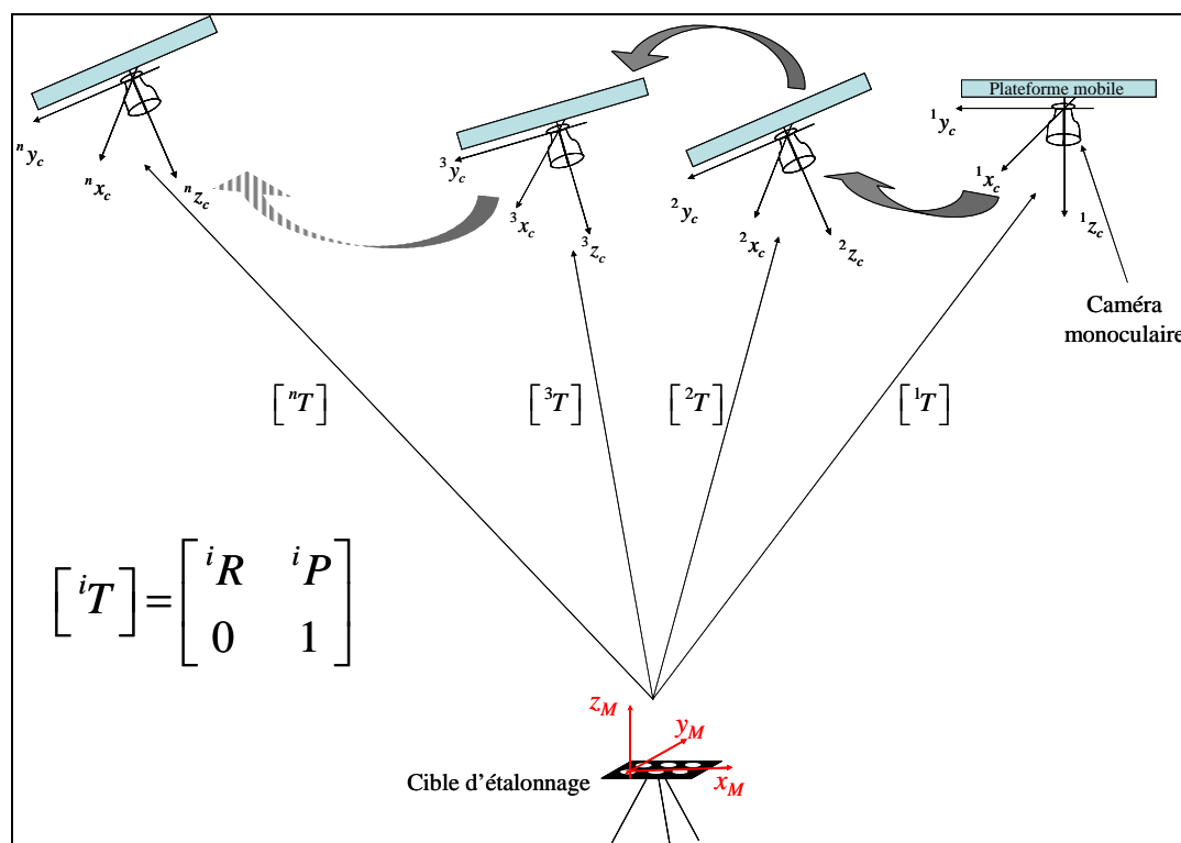
Figure 6-6 : Mesure avec la caméra monoculaire
