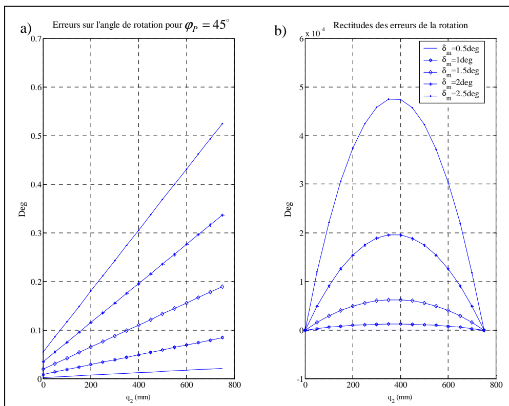
Figure 2-7 : Erreurs e_{\varphi_p} pour \varphi_p = 45^\circ (a) et leurs rectitudes (b)
