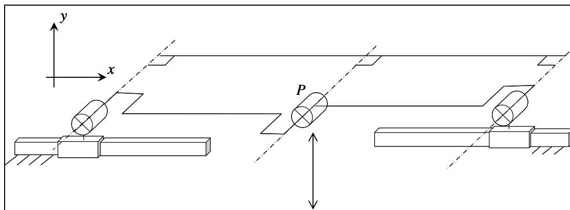
Figure 1-5 : Singularité parallèle
