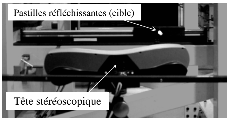
Figure 6-13 : Dispositif de mesure avec la tête stéréoscopique.
