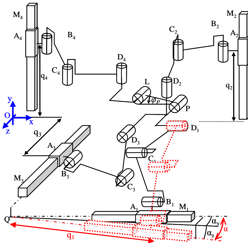
Figure 2-2 : Schéma cinématique de Isoglide4-T3R1 avec défaut d'orientation du moteur M_1
