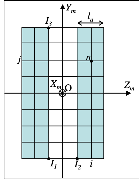
Figure 4-7 : Coordonnées du nœud n dans le repère local
