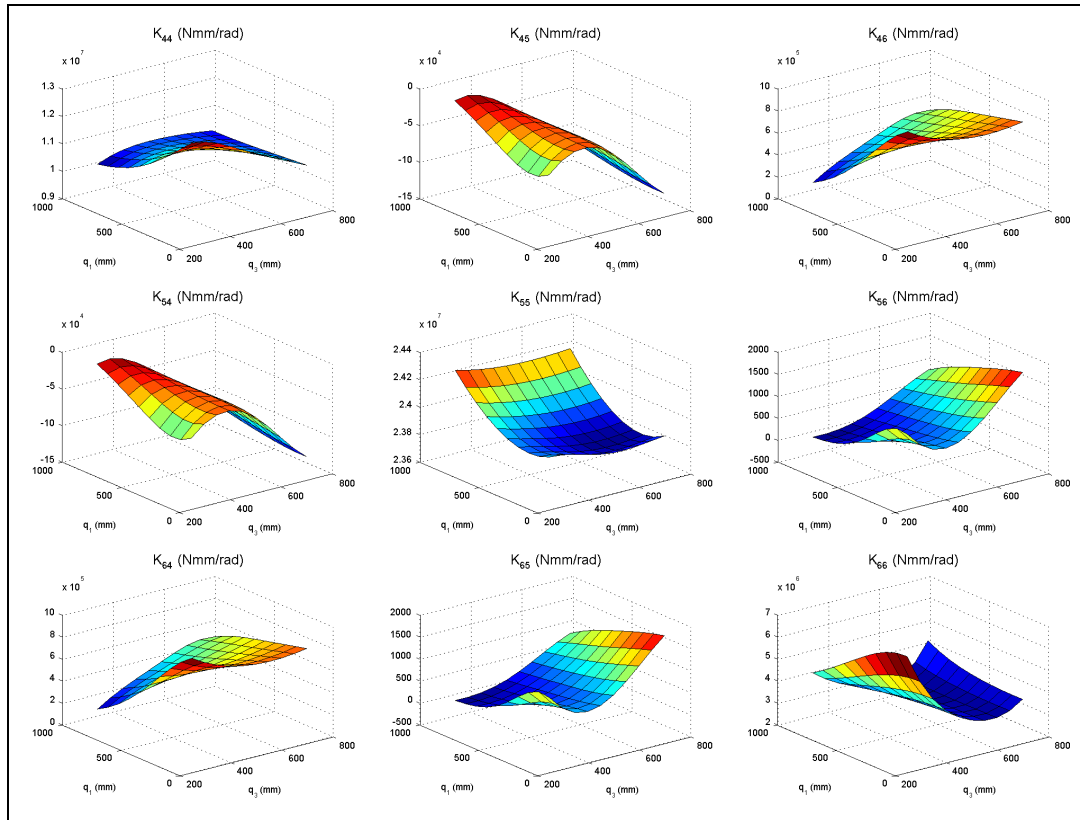
Figure 3-16 : Variations des termes de K_{M0} de l'Isoglide4-T3R1 dans son espace de travail pour q_2=700\text{mm}
