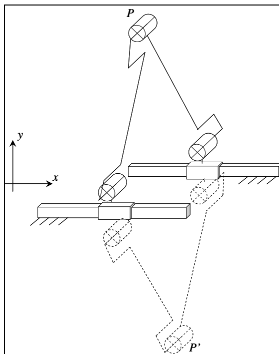
Figure 1-10 : Modes d'assemblage
