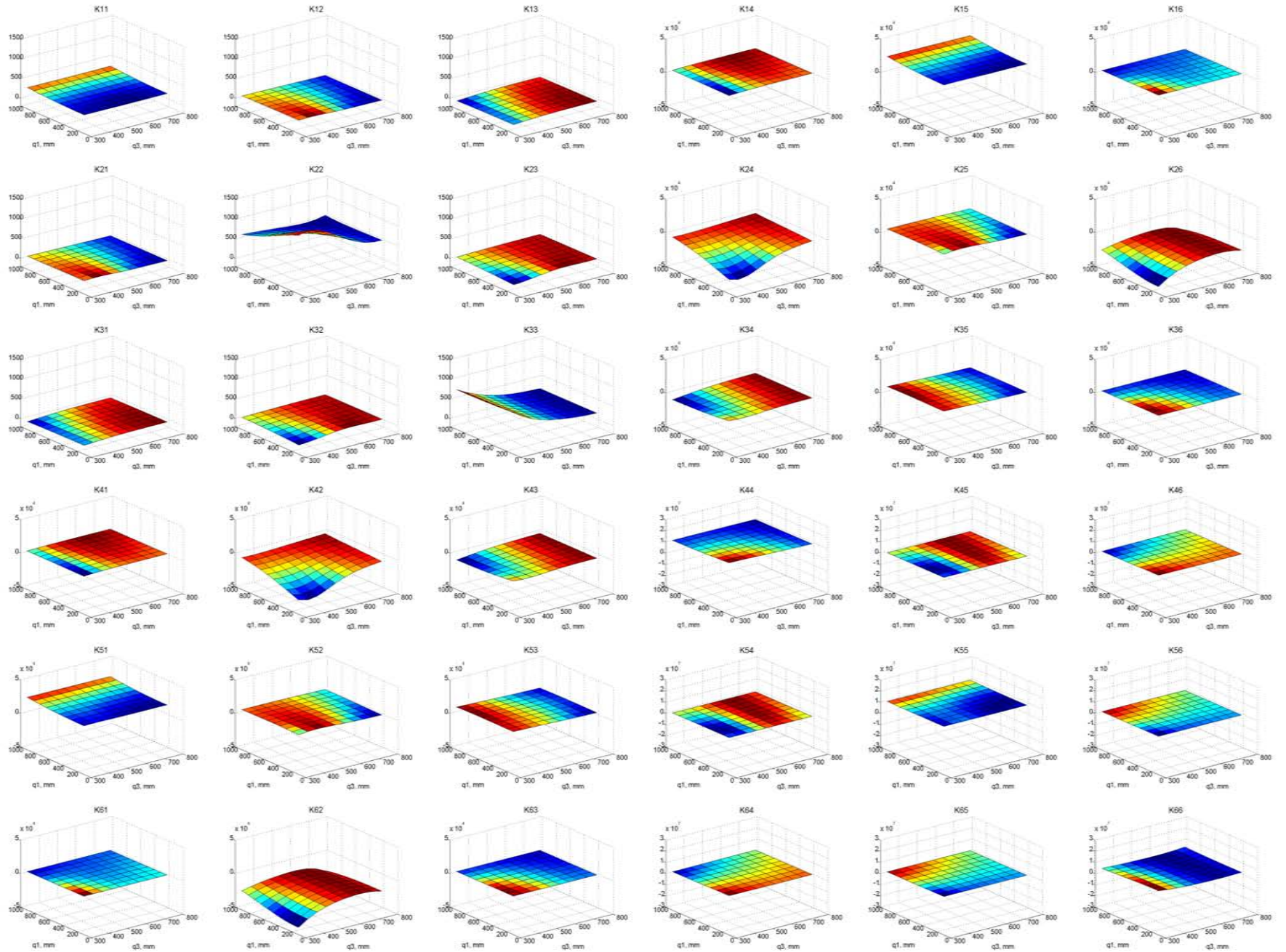
Cartes de rigidité de l'isoglide4-T3R1 condensée à son point caractéristique P pour q_2 = 250 \text{ mm} \varphi_P = 22.5^\circ
