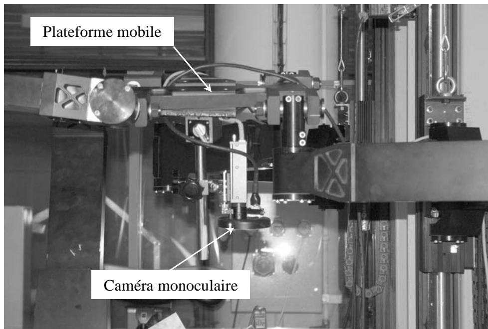
Figure 6-5 : Caméra monoculaire monté en corps rigide sur la plate-forme mobile de l'Isoglide4-T3R1
