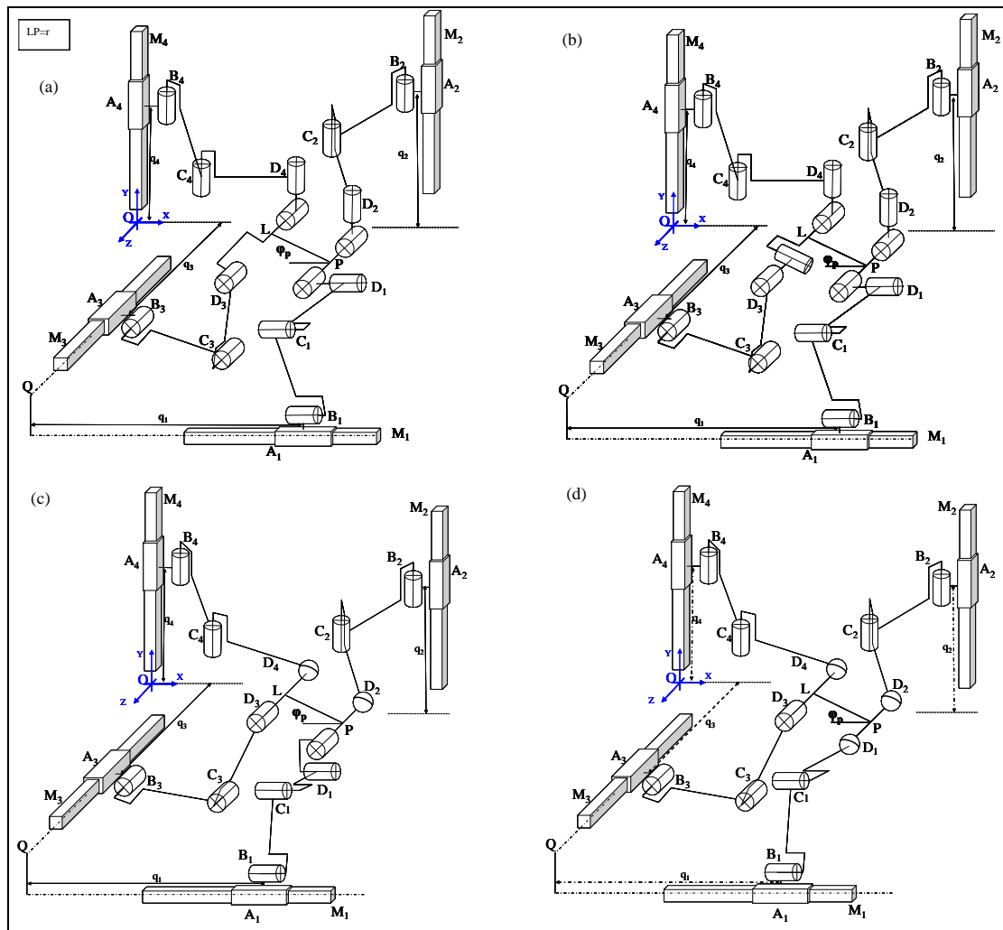
Figure 5-2 : Schémas cinématiques pour quatre versions de l'Isoglide4-T3R1 avec des degrés d'hyperstaticité N=3 (a), N=2 (b), N=1 (c) N=0 (d).
