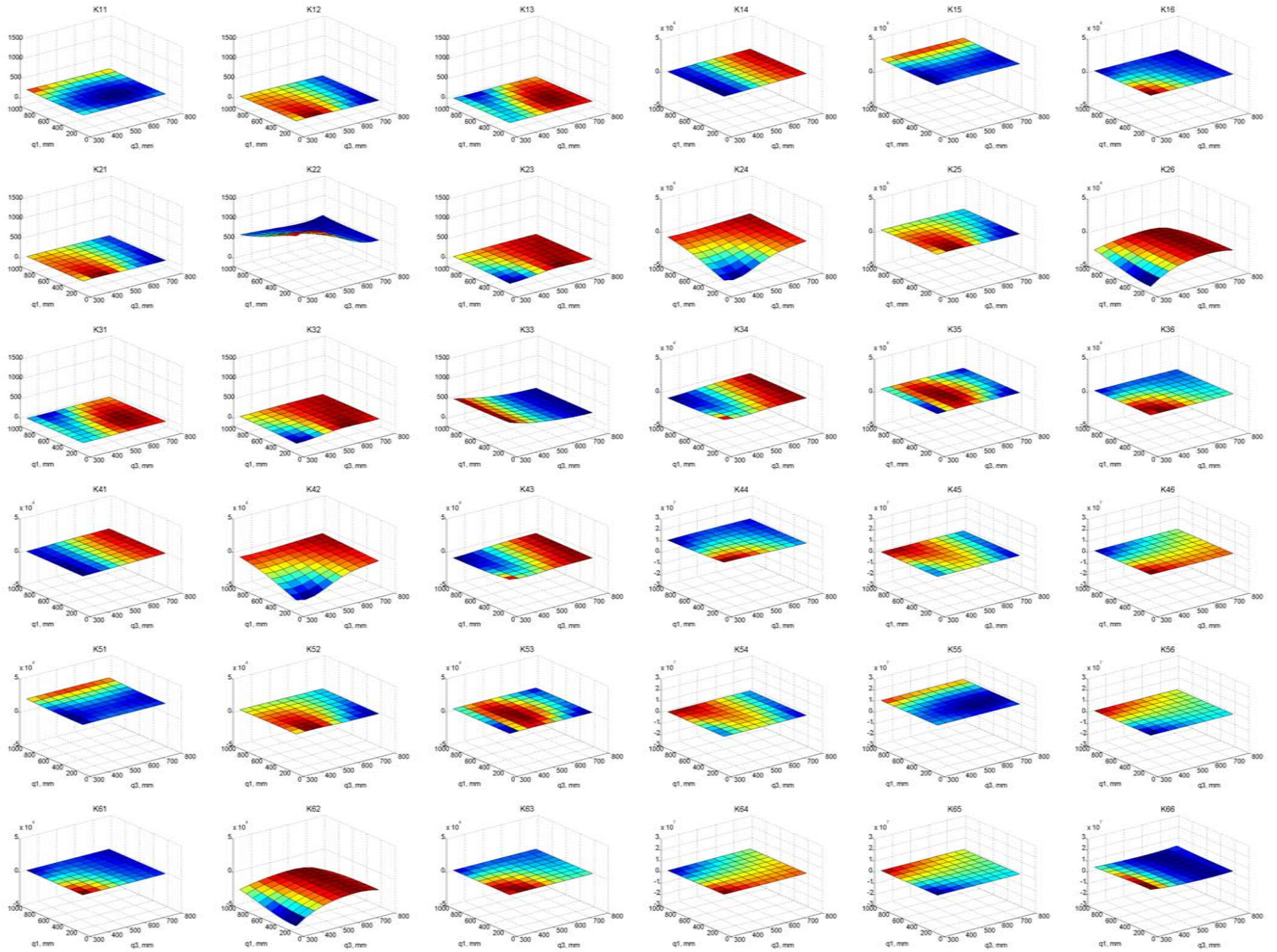
Cartes de rigidité de l'isoglide4-T3R1 condensée à son point caractéristique P pour q_2 = 550 mm \varphi_P = 22.5^\circ
