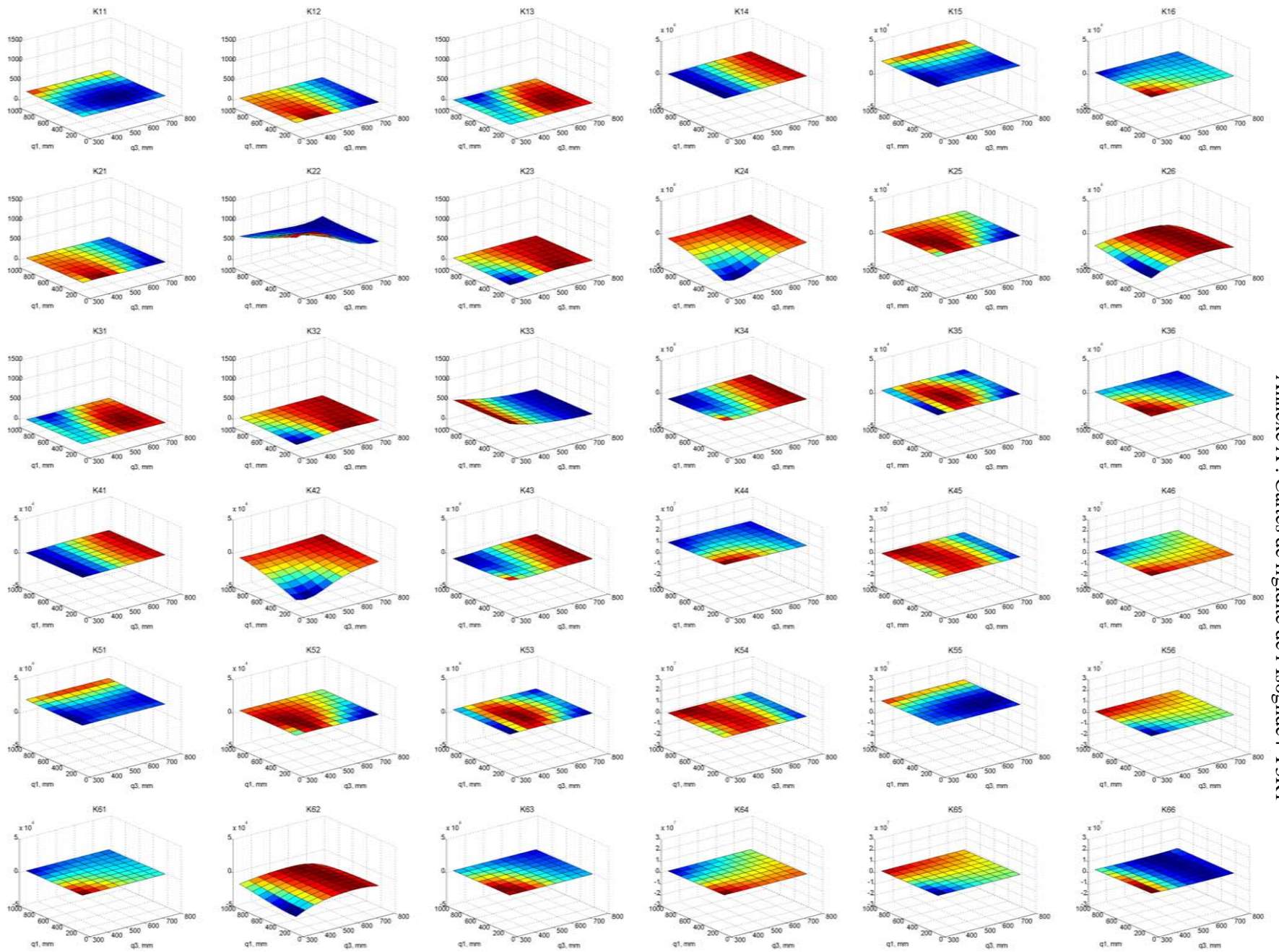
Cartes de rigidité de l'isoglide4-T3R1 condensée à son point caractéristique P pour q_2 = 550 \text{ mm} \varphi_P = 45^\circ
