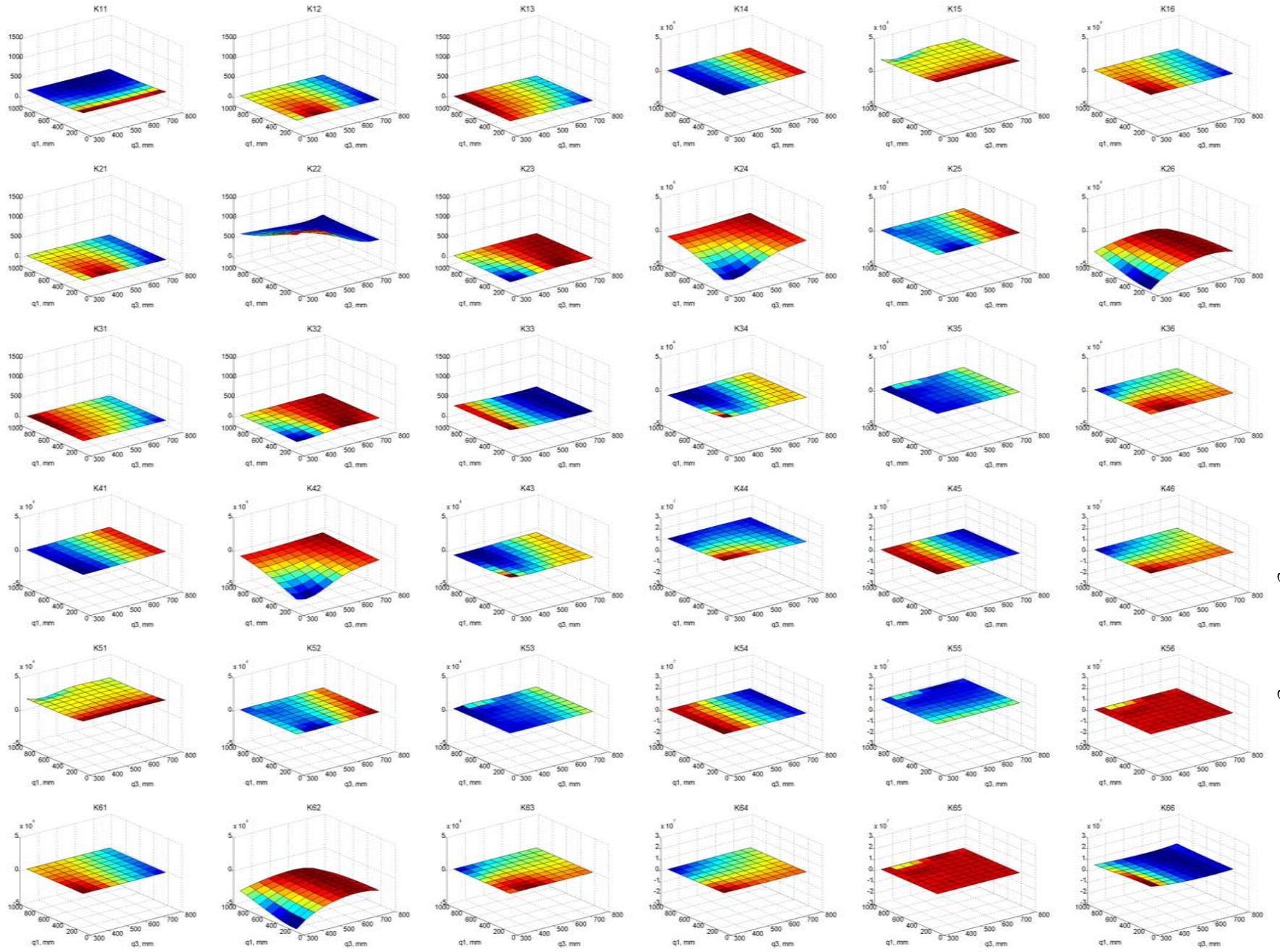
Cartes de rigidité de l'isoglide4-T3R1 condensée à son point caractéristique P pour q_2 = 850 mm \varphi_P = 0^\circ
