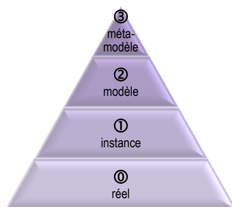
Figure 87 : Les quatre niveaux de modélisation de l'IDM. Figure 88 : Nos quatre niveaux de modélisation.
