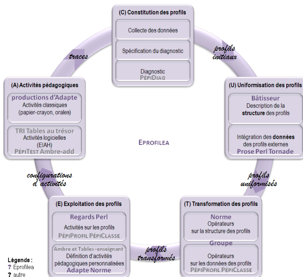
Figure 85 : ACUTE4profiles et l'environnement que nous proposons.
