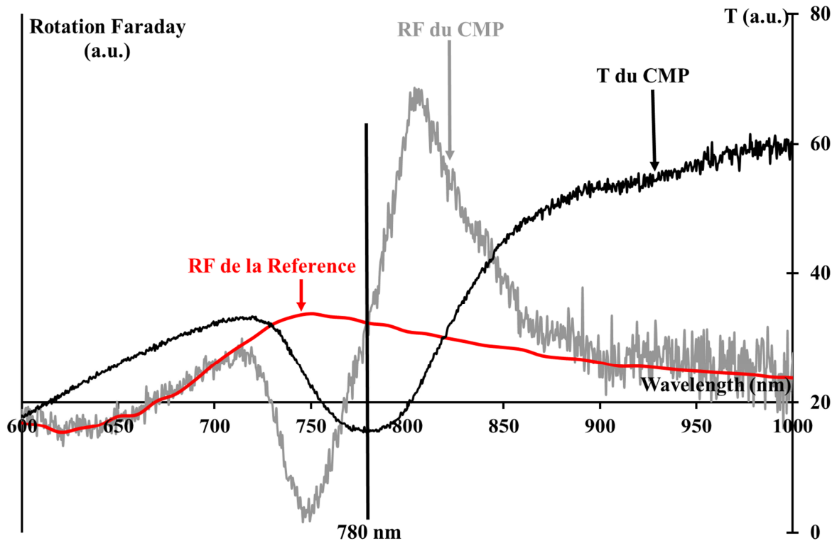
Figure 8.: Les spectres de Transmittance et de rotation de Faraday d'une opale dopée inversée basé sur un template 453 nm, et le spectre de rotation de Faraday d'une monocouche de cobalt-ferrite comme une référence
