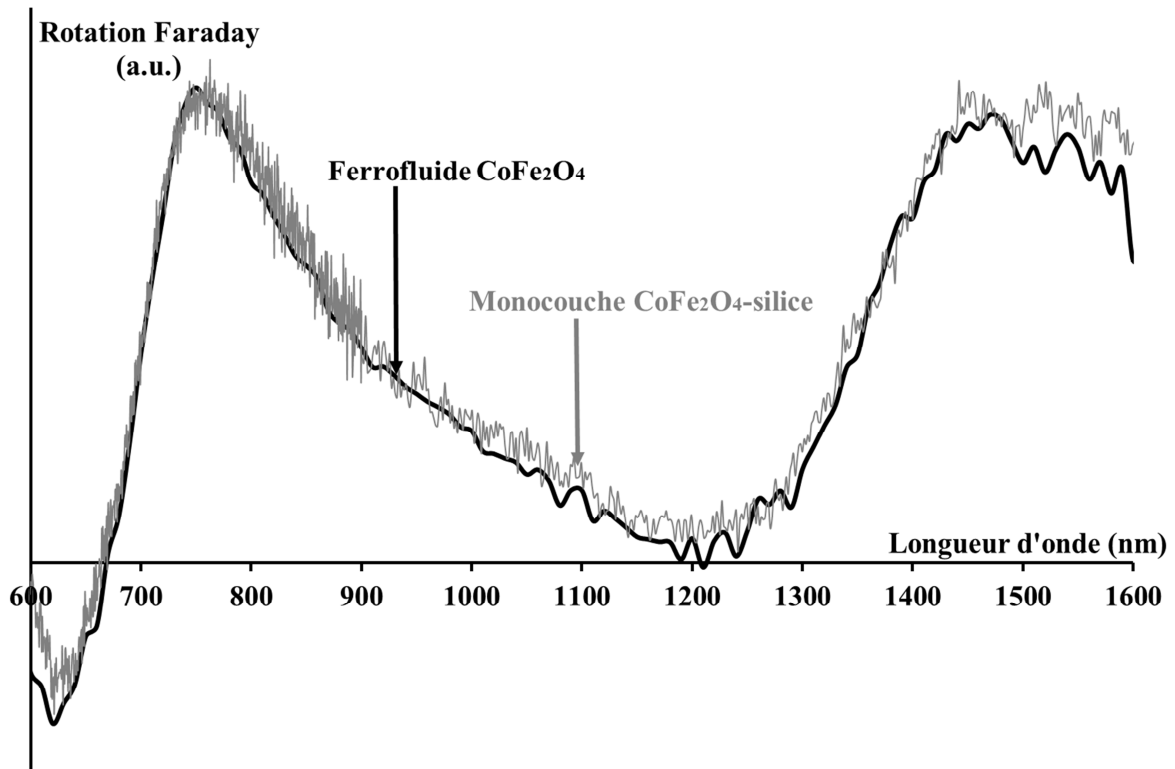
Figure 3.: Les courbes normalisées de rotation de Faraday de la monocouche de silice dopée par \text{CoFe}_2\text{O}_4 et le ferrofluide \text{CoFe}_2\text{O}_4 en fonction de la longueur d'onde
