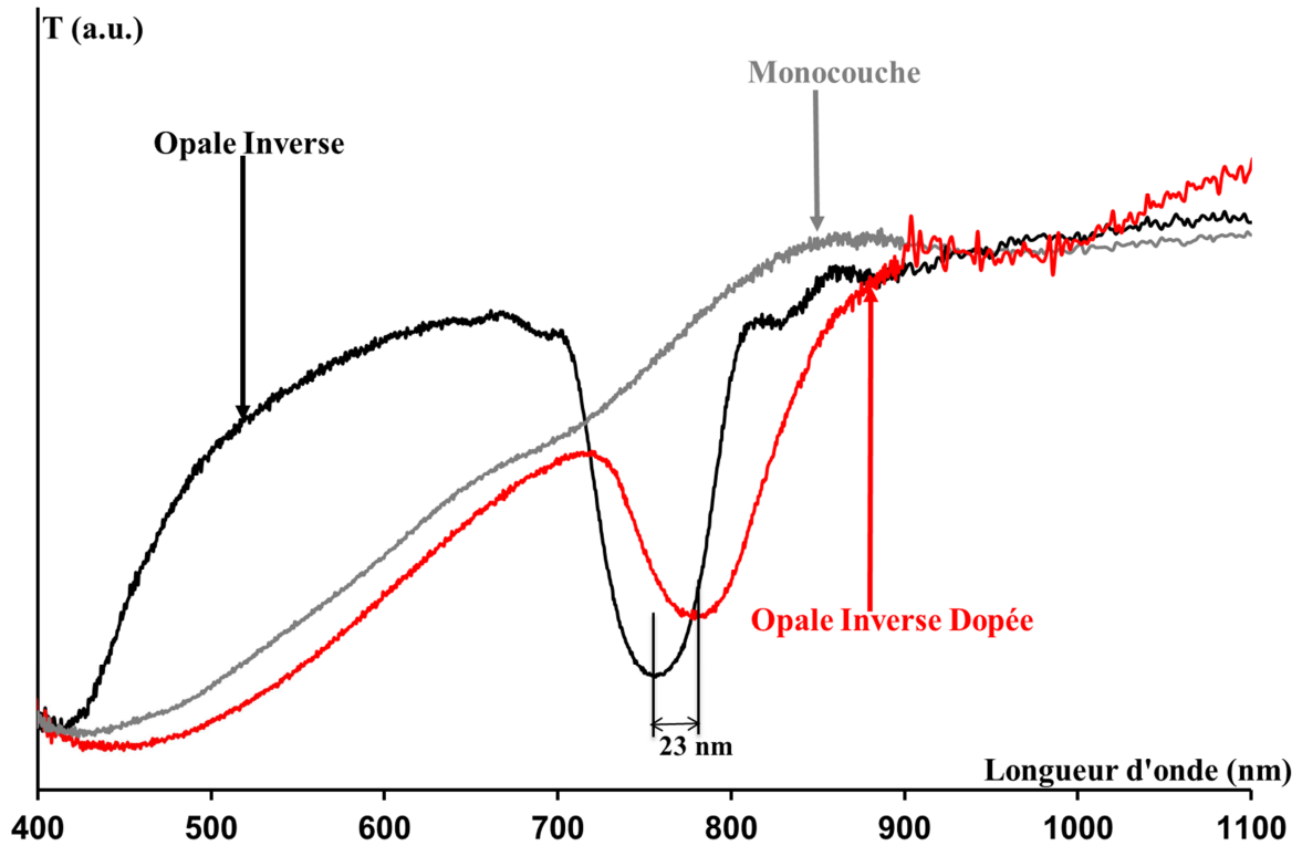
Figure 6.: Mesure de transmittance de la monocouche \text{CoFe}_2\text{O}_4 (monocouche 2:2), d'opale non-magnétiques et magnétiques inverses en fonction de la longueur d'onde (453 nm de taille d_{sph} )
