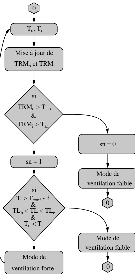
Figure 4.3 – Algorithme du contrôle adaptatif
