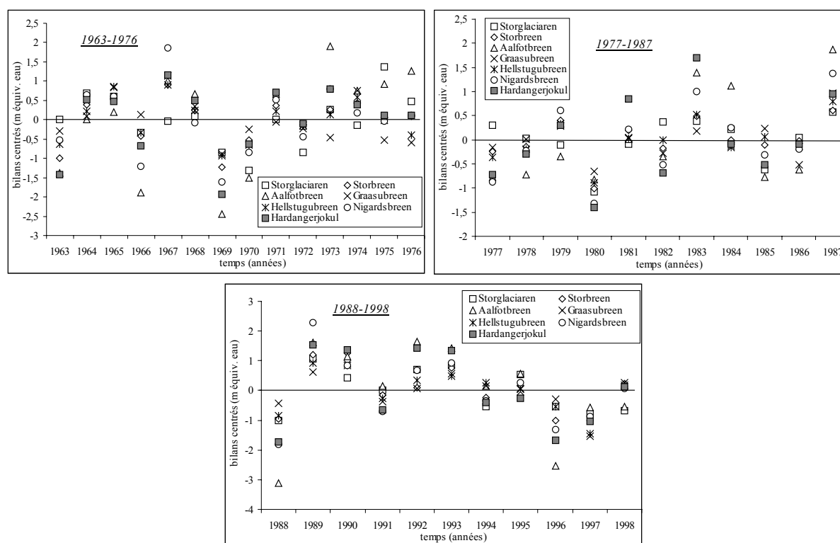
Figure IV.17 : bilans annuels centrés des 7 glaciers scandinaves sur les trois périodes 1963-1976, 1977-1987, 1988-1998 (m equiv. eau)
