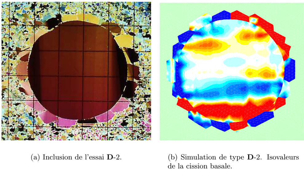
Fig. 7.15 : Comparaison de l'essai D-2 et de la simulation pour une déformation macroscopique de 5.8%.
