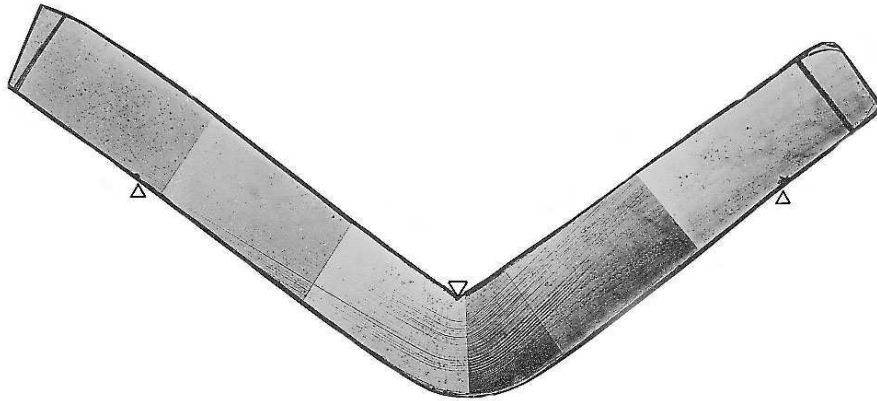
(a) Photographie de l'échantillon 266 de Nakaya (1958).
