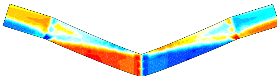
(b) Simulation avec orientations continues, \alpha = 1 , \beta = 0.01 .
