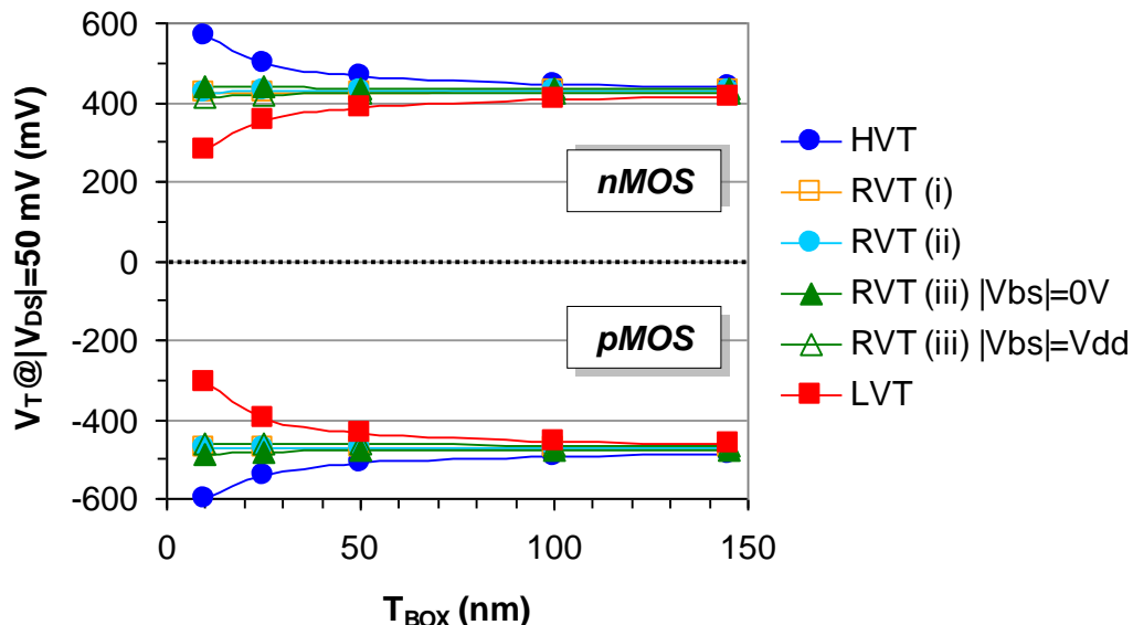
Figure 4.10. : Evolution de la tension de seuil ( V_T ) en régime linéaire ( |V_{DS}|=50 \text{ mV} ) en fonction de T_{BOX} pour plusieurs configurations de BP d'un transistor nMOS et d'un transistor pMOS FDSOI à canal long ( L_G=1 \mu m ) et ayant un film mince de silicium non dopé d'une épaisseur T_{Si}=6 \text{ nm} , un oxyde de grille avant d'une épaisseur T_{OX}=1,2 et une tension d'alimentation V_{DD}=0,9 \text{ V} .
