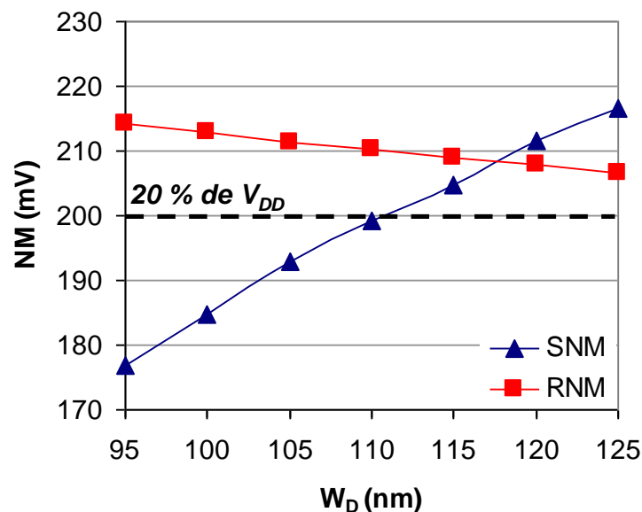
Figure 7.19. : Evolution de la marge de bruit en lecture (SNM) et en rétention (RNM) en fonction de W_D de la cellule SRAM 4T LL FDSOI simulée dans le nœud technologique 45 nm.
