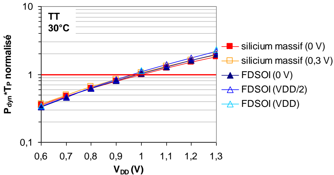
Figure 7.4. : Evolution du produit P_{\text{dyn}} \cdot \tau_P normalisé en fonction de V_{\text{DD}} du chemin critique simulé avec une carte modèle silicium massif basse consommation (carré) et FDSOI (triangle) dans le nœud technologique 28 nm.
