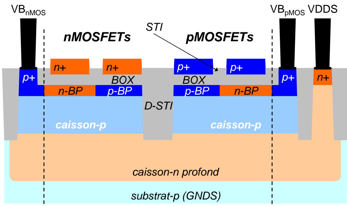
Figure 6.10. : Vue en coupe schématique d'une cellule standard multi- V_T FDSOI basée sur le schéma d'intégration spécifique avec isolation latérale des caissons-p par D-STI.
