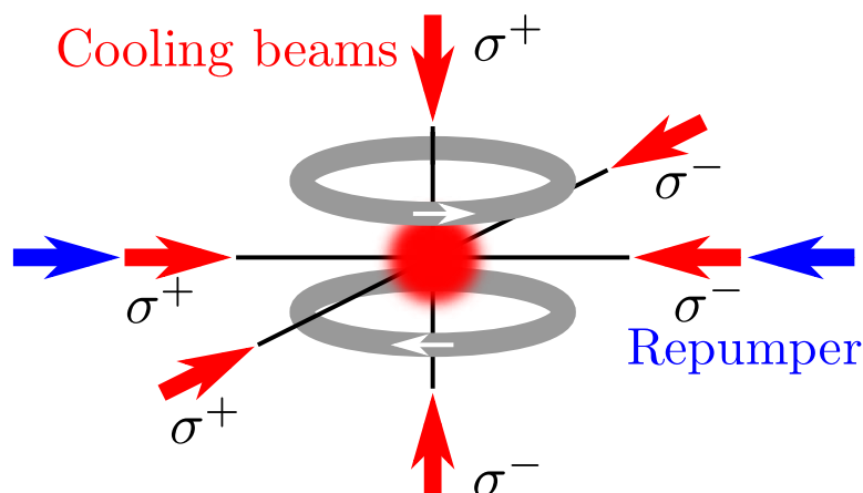
Figure 2.1 – Géométrie du piège magnéto-optique. Le champ magnétique quadrupolaire est généré par une paire de bobines en configuration anti-Helmoltz. Six faisceaux laser polarisés circulairement, désaccordés dans le rouge (flèches rouges) et deux faisceaux repompeurs (flèches bleues) sont alignés sur le centre du piège.
