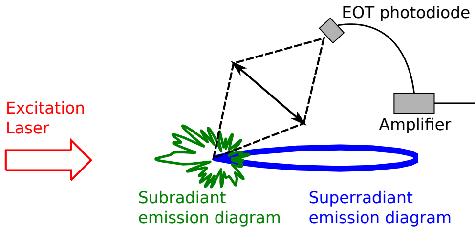
Figure 2.13 – Dispositif expérimental pour l’observation de la sousradiance.
