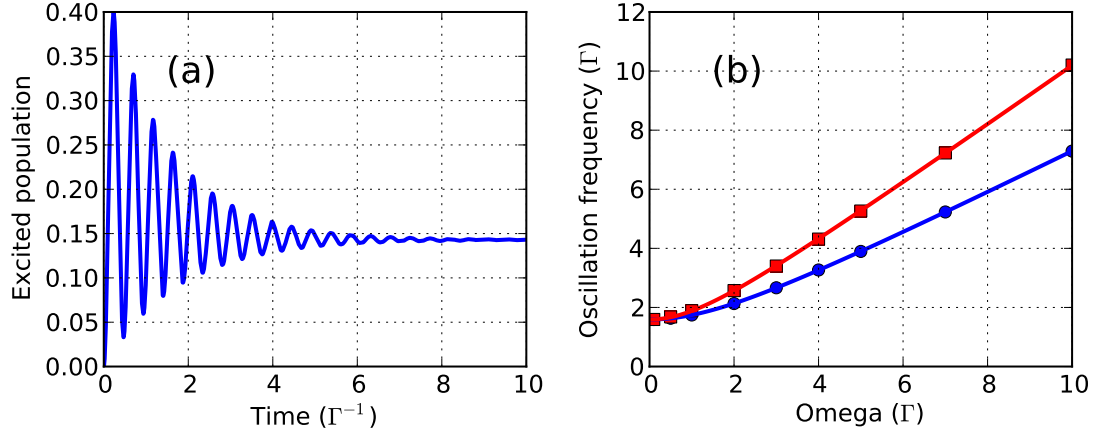
Figure 1.8 – (a) Population des états excités en fonction du temps. Les atomes sont initialement dans l'état fondamental |G\rangle et le laser est allumé à t = 0 . On observe des oscillations de Rabi amorties. Paramètres de la simulation : N = 40 , k\sigma = 10 , \Delta = 10\Gamma , \Omega = 2\Gamma . (b) Fréquences d'oscillation de la population des états excités en fonction de \Omega pour N = 20 (cercles bleus) et N = 40 (carrés rouges) ainsi que leurs prédictions théoriques sans ajustement f_R = \sqrt{N\Omega^2 + \Delta^2}/(2\pi) (courbes continues).
