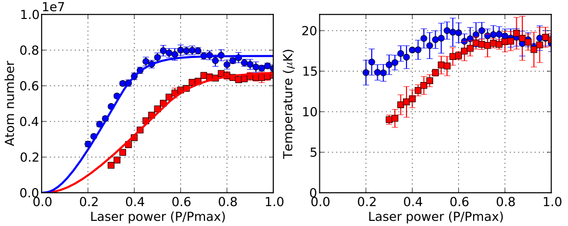
Figure 3.12 – Nombre d’atomes et température des atomes dans le piège dipolaire, 60 ms après le chargement, en fonction de la puissance laser ( P_{\max} = 200 mW) pour un désaccord de \Delta = 20 GHz (cercles bleus) et \Delta = 40 GHz (carrés rouges). Les courbes en traits pleins sur la figure de gauche correspondent aux ajustements à partir de la formule 3.22. Paramètres : L = 1 mm, w = 65 \mu\text{m} , f_m = 90 kHz.
