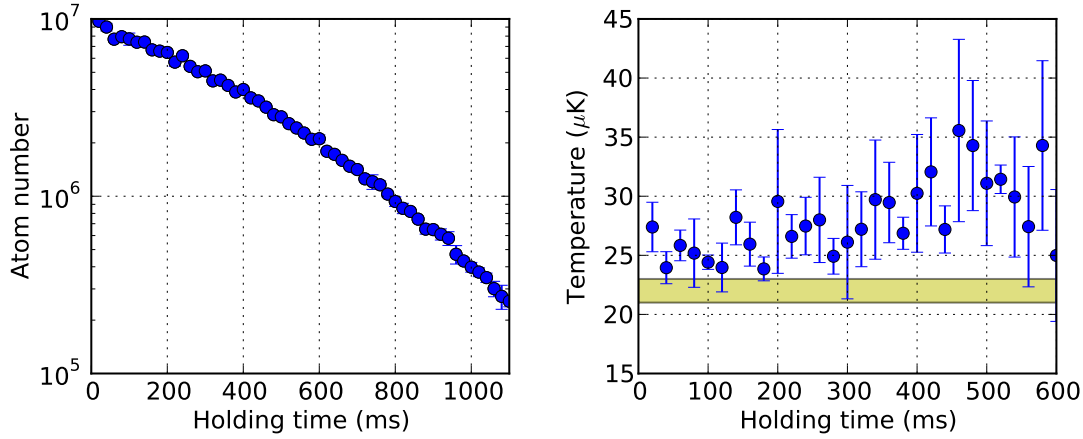
Figure 3.21 – Nombre d’atomes et température du nuage piégé en fonction du temps de maintien pour les paramètres suivants : P = 200 \text{ mW} , \Delta = 40 \text{ GHz} , L = 1 \text{ mm} , w = 65 \mu\text{m} , f_m = 90 \text{ kHz} . Un ajustement sur les premières 500 ms de la courbe donne un temps de vie de 442 ms. La zone colorée correspond à la température initiale du dark MOT ( 22 \mu\text{K} ) avant le chargement du piège dipolaire bleu.
