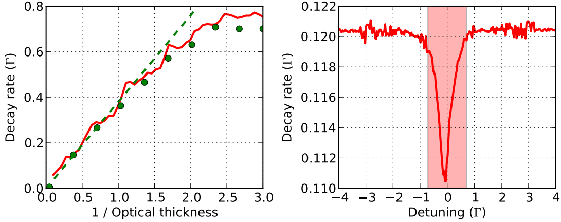
Figure 1.15 – La figure de gauche donne le taux d'émission sous-radiant en fonction de 1/b_0 . Nous avons gardé le nombre d'atomes N = 400 et le désaccord \Delta = 10\Gamma constants et nous avons fait varier la taille du système k\sigma . La courbe rouge correspond au taux de relaxation sous-radiant mesuré sur les courbes de relaxation temporelle. Pour de grandes épaisseurs optiques, le taux d'émission est proportionnel à \Gamma/b_0 (cf. courbe en pointillés verts) et tend vers \Gamma pour les nuages dilués. Les cercles verts correspondent aux taux de relaxation du mode de la matrice \mathcal{H} (Eq.(1.160)) ayant le plus grand temps de vie. On remarque le très bon accord entre l'approche de la relaxation temporelle du système et l'étude des modes de la matrice \mathcal{H} . La figure de droite montre le taux d'émission sous-radiant en fonction du désaccord pour b_0 = 3 ( N = 400 , k\sigma = 20 ). La région colorée correspond à la région de diffusion multiple b(\Delta) > 1 .
