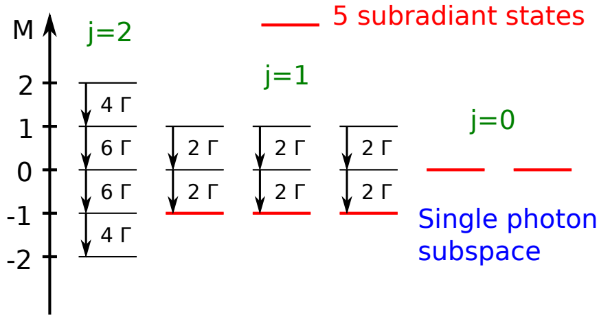
Figure 1.7 – Décomposition de l’espace de Hilbert pour un système de quatre atomes à deux niveaux en somme d’espaces propres de \{S^2, S_z\} (voir Eq. 1.94). Les taux d’émission spontanée entre états sont donnés par l’équation (1.93). Les cinq états sousradiants sont représentés en rouge. La région bleutée représente le sous-espace de Hilbert engendré par |G\rangle et les états à une excitation. C’est dans cet espace que nous étudions les effets coopératifs.
