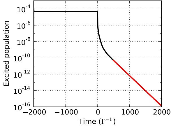
Figure 1.14 – Population des états excités en fonction du temps pour les mêmes paramètres que ceux de la figure 1.12 : N = 2000 , k\sigma = 10 , \Omega = 0.01\Gamma , \Delta = 10\Gamma . Le laser est éteint à t = 0 . Cette courbe et la figure 1.12 mettent en évidence que la sousradiance n’a une décroissance purement exponentielle qu’après un certain temps (partie rouge de la courbe). Cela se produit lorsque le mode avec le plus grand temps de vie domine. Le taux de relaxation associé à ce régime est appelé taux de relaxation sousradiant \Gamma_{\text{sub}} . Dans cet exemple, ce dernier vaut 8.5 \cdot 10^{-3}\Gamma .
