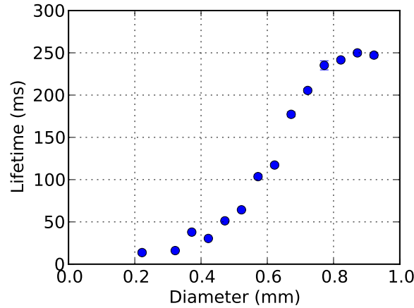
Figure 3.15 – Temps de vie du nuage en fonction du diamètre du piège. Paramètres : P = 200 \text{ mW} , \Delta = 40 \text{ GHz} , w = 65 \mu\text{m} , f_m = 90 \text{ kHz} .
