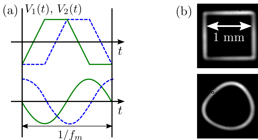
Figure 3.6 – Image d'une coupe transverse d'un tube du piège pour deux types de modulation différents. À titre d'exemple, nous montrons deux configurations utiles en pratique. (a) Signaux électriques ( V_1(t) , V_2(t) ) envoyés aux VCOs. (b) Images des coupes transverses. La taille du piège est de L = 1.05 mm pour un waist de w = 65 \mu m.
