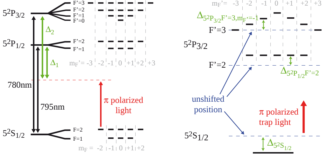
Figure C.1 – Déplacement lumineux pour les niveaux du ^{87}\text{Rb} pour une lumière polarisée \pi . L'état initial du système est |g\rangle \equiv |5^2S_{1/2}, F = 2, m_F = 0, \pm 1, \pm 2\rangle . La figure de gauche montre les différents niveaux excités couplés par le laser. Dans notre situation, on peut négliger les transitions de la raie D_1 et considérer un même désaccord pour tous les niveaux de la raie D_2 . La figure de droite illustre les déplacements des niveaux hyperfins |5^2P_{3/2}, F' = 2, m_{F'}\rangle et |5^2P_{3/2}, F' = 3, m_{F'}\rangle . Figure tirée de [45].
