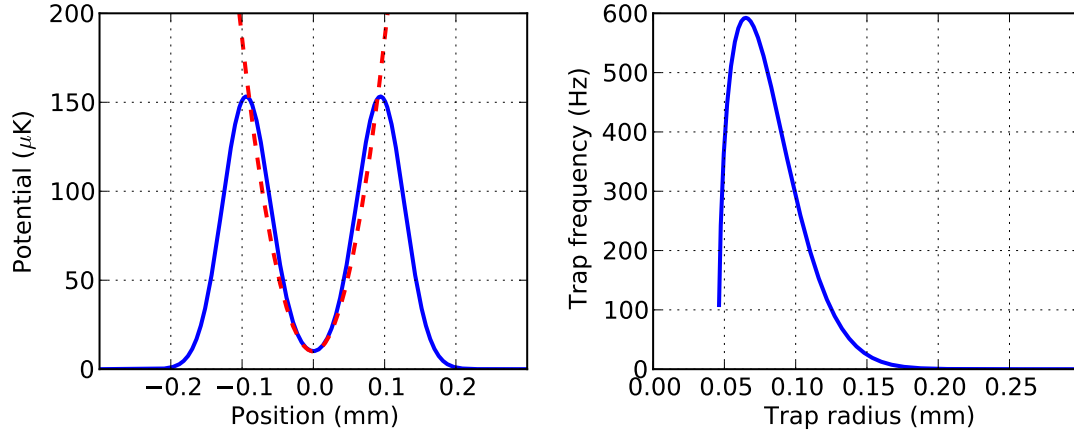
Figure 3.5 – La figure de gauche montre le potentiel dipolaire et son approximation harmonique donnée par l'équation (3.15). Paramètres utilisés : P = 2\text{W} , désaccord 8\text{ nm} , a = 100\ \mu\text{m} , w = 65\ \mu\text{m} . La fréquence du piège est de \omega/2\pi = 290\text{ Hz} . La figure de droite montre l'évolution de la fréquence du piège harmonique en fonction du rayon du piège.
