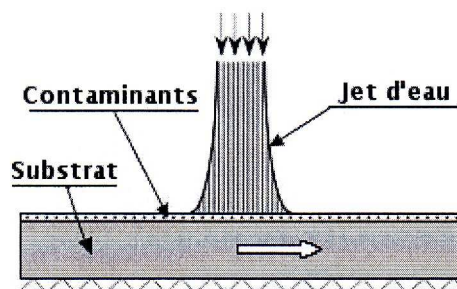
Figure 1.8. Schéma du décapage par jet d'eau [34]
