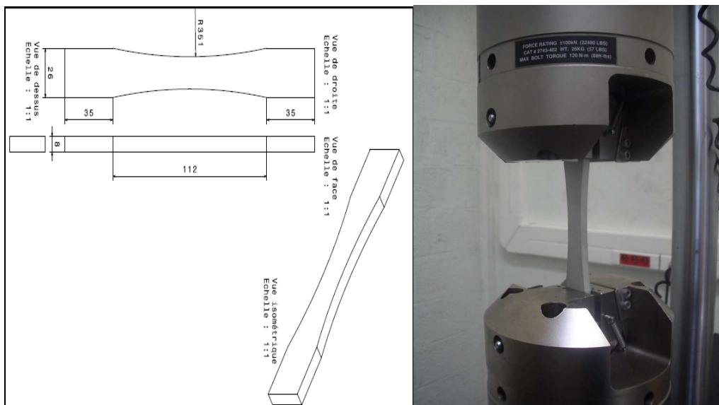
Figure 2.12. Dispositif expérimental (a) croquis des éprouvettes de fatigue [17], (b) représentation du montage d'une éprouvette sur machine
