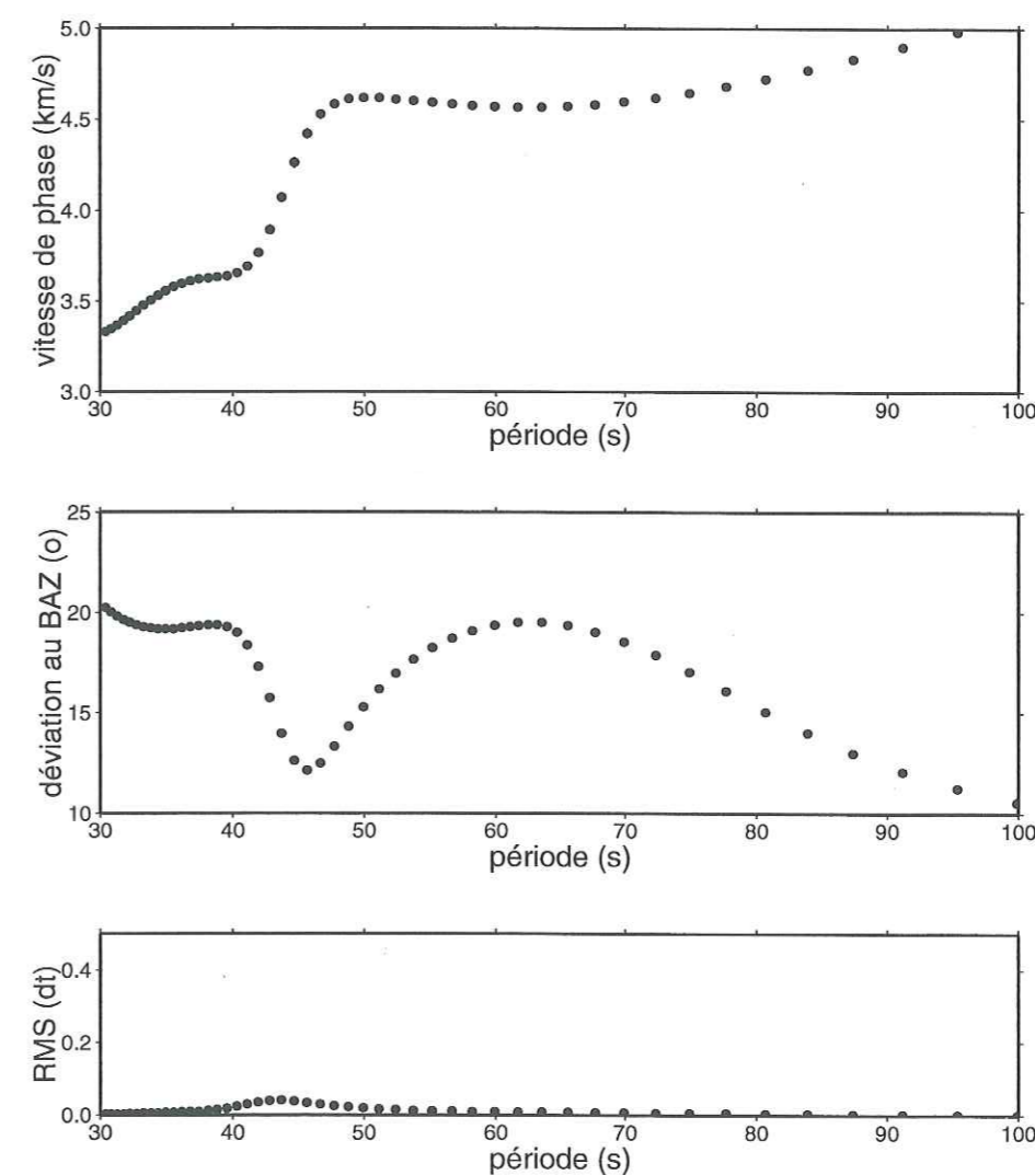
FIG. 1.11 – Résultats de l'analyse en fréquence du séisme du Pérou (12 novembre 1996) pour la composante verticale. La mesure apparaît instable entre 40 et 55 secondes de période pour lesquelles le rms augmente. Ceci est dû au fait que dans le signal d'origine le spectre en amplitude présente un trou entre ces périodes et le rapport signal/bruit est alors petit (inférieur à 1.5) pour obtenir une mesure stable.
