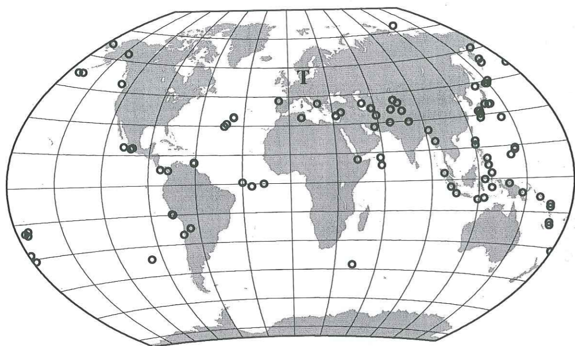
FIG. 6.6 – Carte mondiale représentant la répartition des épicesentres des 99 événements sélectionnés pour notre étude. La répartition spatiale étendue permet d'avoir une bonne couverture azimutale et une bonne répartition épicesentrale. La lettre T situe la région étudiée.
