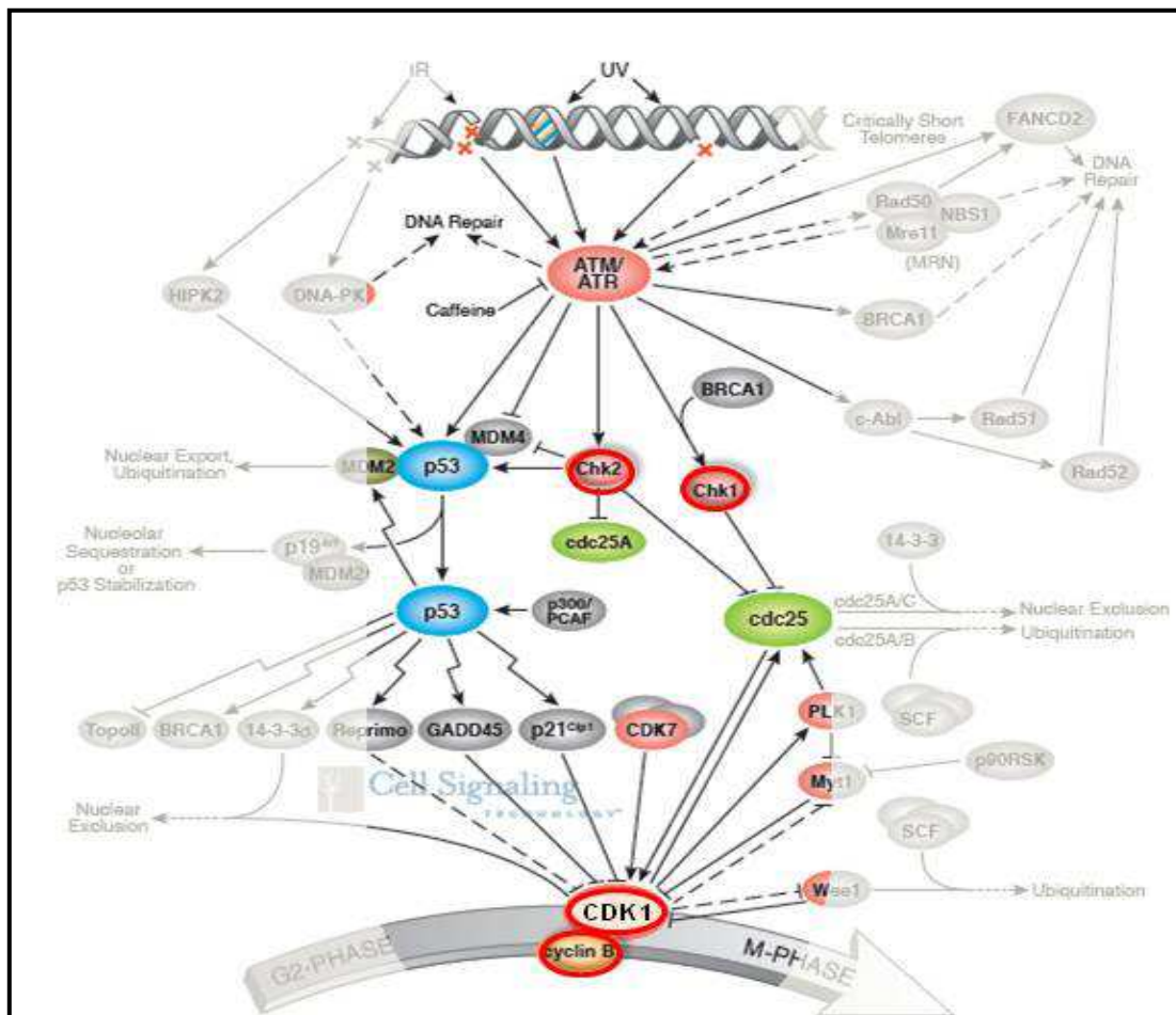
Figure 28: Modèle d'arrêt du cycle en phase G2/M suite au traitement des cellules au S23906-1 (d'après Cell Signaling Technology ). L'induction de lésions à l'ADN par le S23906-1 active Chk2 qui va ensuite indirectement inhiber le complexe cycline B/Cdk1.
