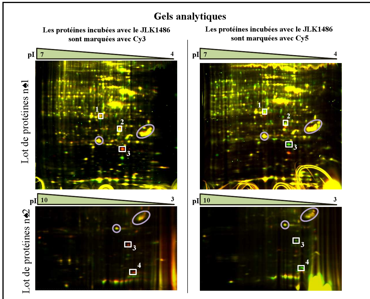
Figure 94: Electrophorèse 2D-DIGE des protéines incubées ou non avec le JLK1486. Les expériences sont réalisées en triplicate pour chacun des lots protéiques. Les protéines fluorescentes du lot n°1, incubées ou non avec le JLK1486, ont été déposées sur des strips 4-7 et la seconde dimension a été réalisée sur un gel d'acrylamide 8-16%. Les protéines fluorescentes du lot n°2, incubées ou non avec le JLK1486, ont été quant à elle déposées sur des strips 3-10 et la seconde dimension a été réalisées sur un gel d'acrylamide 9-15%. Les cercles sont des références et permettent de comparer les gels entre eux. Le différentiel de fluorescence observé au niveau des spots 3 et 4 montrent déjà une interaction potentielle entre les protéines contenues dans celui-ci et le JLK1486. L'analyse des gels par le logiciel SameSpot a ensuite mis en évidence deux autres spots intéressants. Le spot 3 est retrouvé sur les gels des deux lots de protéines.
