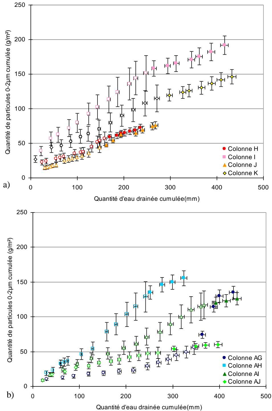
Figure 4.15 : Evolution des quantités cumulées de particules exportées en fonction des quantités d'eau drainée cumulée pour chaque colonne de l'expérimentation L1. a) Intensité 20 mm/h b) Intensité 6 mm/h. Les figurés vides représentent les concentrations estimées et les figurés pleins les concentrations mesurées
