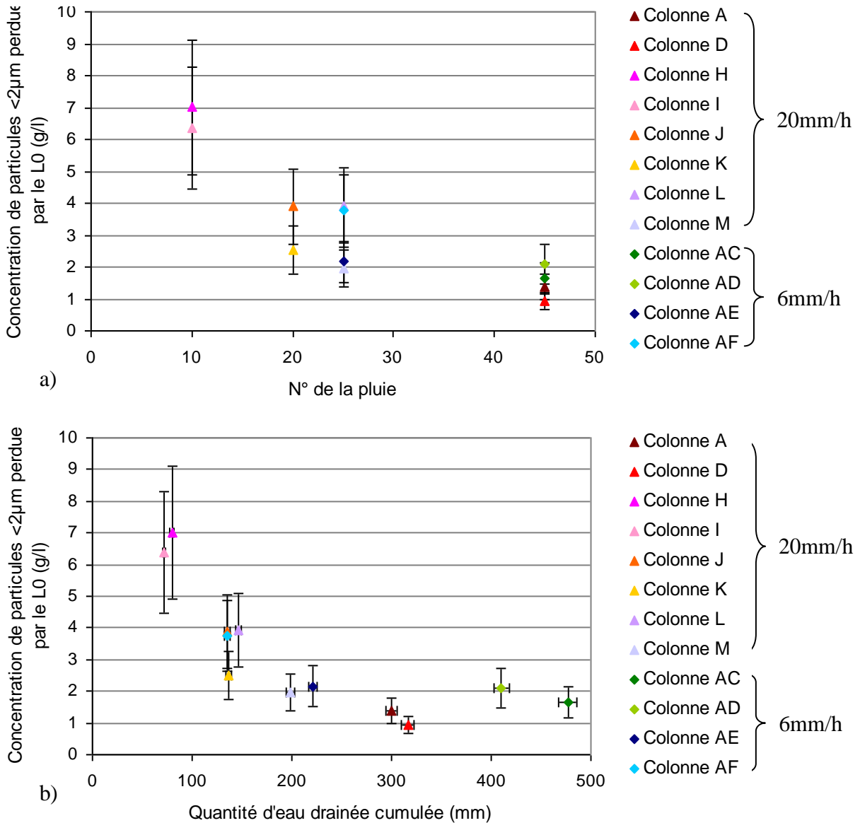
Figure 4.5 : Evolution temporelle de la concentration de particules de taille 0-2 µm mesurée à la base des colonnes de sol pour l'expérimentation L0. a) en fonction du numéro de la pluie, b) en fonction du drainage cumulé. Pour mémoire les concentrations de 0-2 µm de L0 dans LQ ont été mesurées par infra-rouge moyen sur différentes couches du LQ et sur les particules collectées dans le bac sous-jacent. Les concentrations présentées dans cette figure résultent d'un calcul de moyenne pondérée sur les différentes couches et le bac
