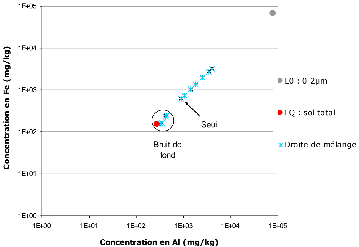
Figure 2.26 : Rapport Fe/Al déterminé par la méthode d'extraction à l'eau régale pour les deux pôles purs 0-2 \mu\text{m} de L0 et sol total de LQ et pour les 11 échantillons standards
