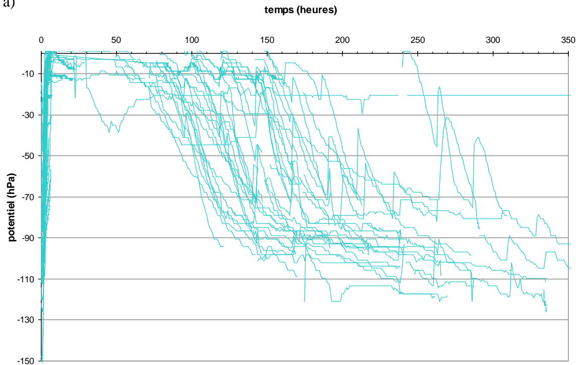
Figure 2.15 : Evolution temporelle du potentiel matriciel au cours des différents cycles « pluie-sécherage » pour le tensiomètre situé à 5 cm dans le LQ pour a) l'intensité 20 mm/h et b) l'intensité 6 mm/h
