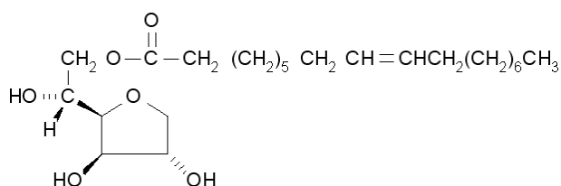
Figure 81 : Molécule de Span 80
