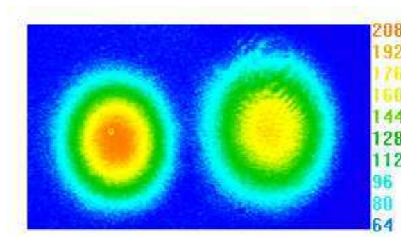
Figure 2.11. Image des deux faisceaux issus de l'interféromètre de Michelson avant la correction de l'alignement avec les deux miroirs fixe et mobile (différentes intensités et différentes tailles pour les deux faisceaux)
