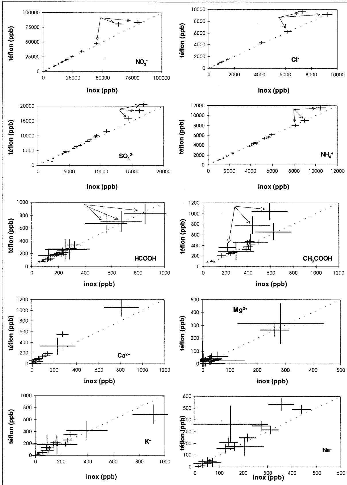
Figure IV.2. : Evaluation de l'influence du support d'impaction par comparaison des concentrations sur les 2 moitiés de la tige mixte inox-téflon.
