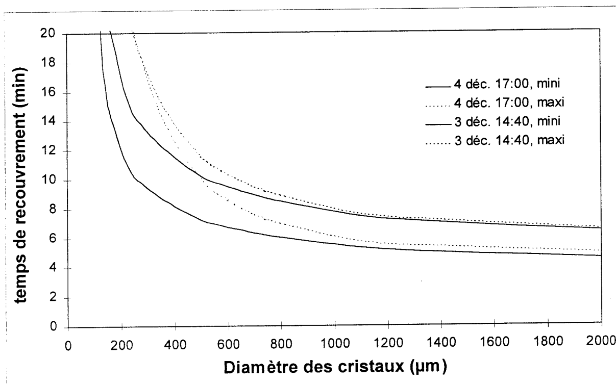
Figure A4.3. : Temps de recouvrement calculés pour 2 cas de neiges des 3 et 4 décembre.
