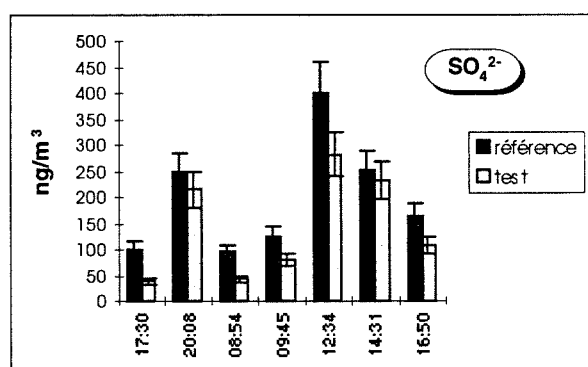
Figure IV.6. : Concentrations de sulfate dans l'aérosol mesuré dans les 2 lignes en parallèle.
