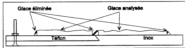
Figure IV.1. : Tige d'impacteur utilisée pour l'étude de l'influence du matériau sur la rétention des solutés.
