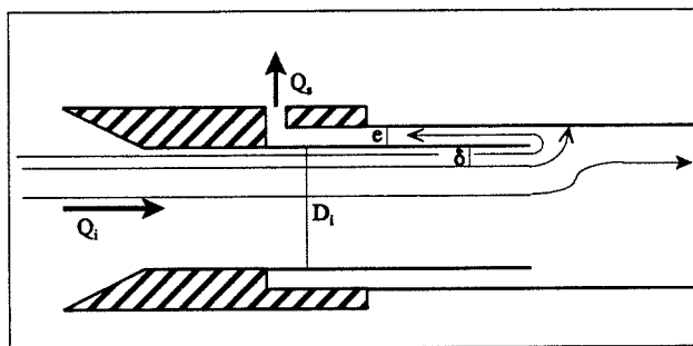
Figure II.2. : Notations et illustration du calcul de dimensionnement du séparateur. Q_i débit principal ; Q_s débit d'échantillonnage ; D_i diamètre du tube intérieur ; e écart entre les 2 tubes coaxiaux ; \delta largeur de la couronne permettant un débit Q_s dans le tube principal.
