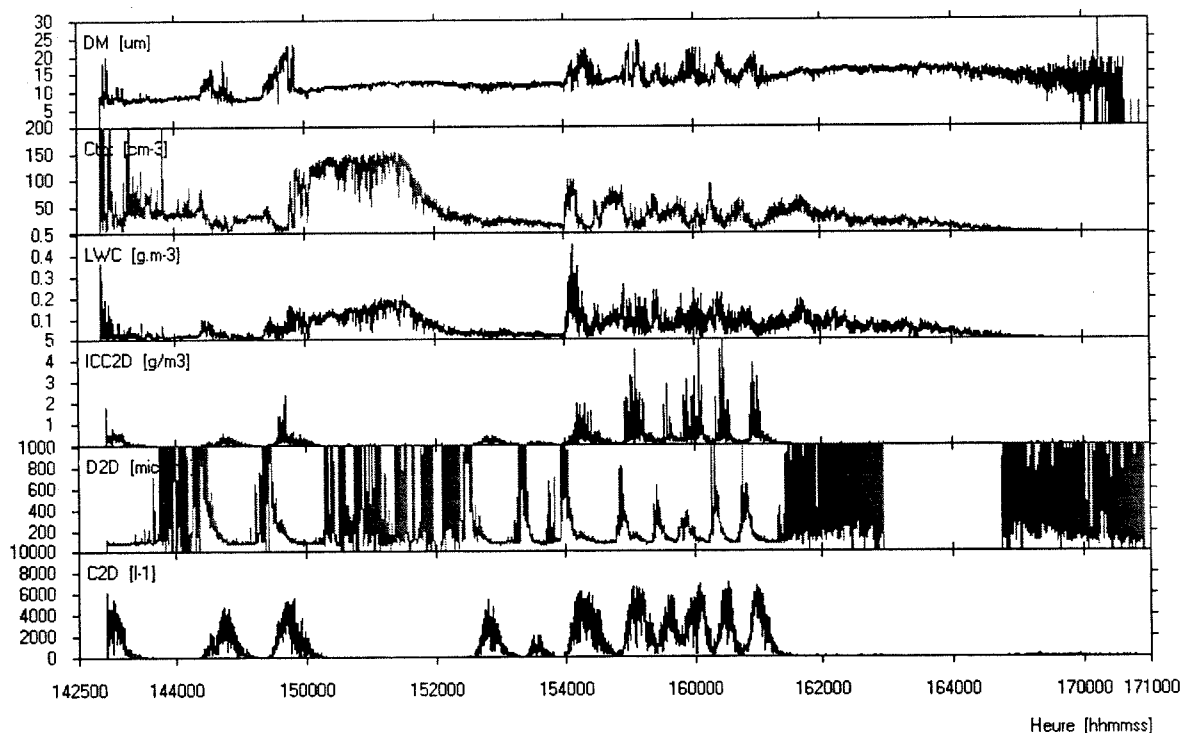
Figure III.2. : Exemple de données de microphysique obtenues pour la journée du 4 décembre. Ces profils sont ensuite moyennés sur la durée des prélèvements chimiques.
