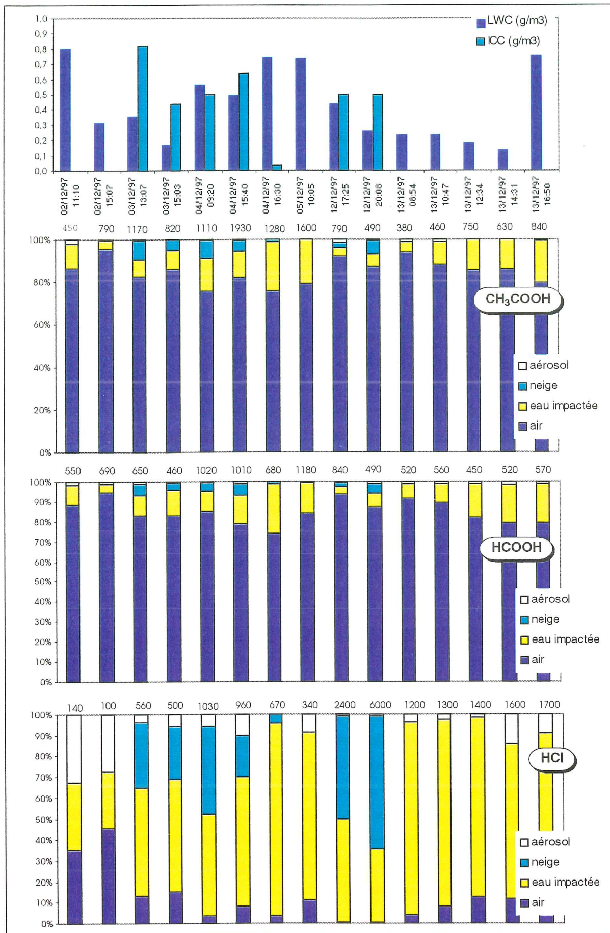
Figure III.7. : Répartition des espèces étudiées entre les différentes phases, en fraction de la masse totale mesurée dans le nuage. Celle-ci est indiquée (ng/m 3 ) en haut de chaque colonne.
