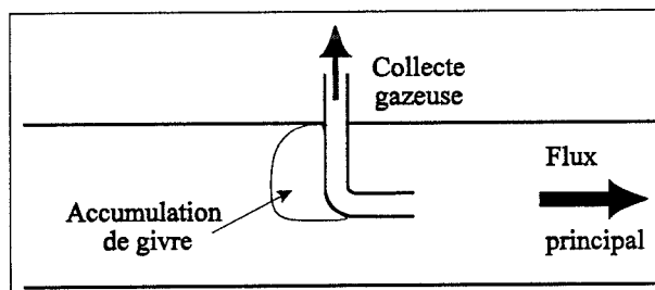
Figure II.1. : Géométrie inadaptée à la collecte dans les nuages froids à cause des risques de réémission de gaz lors du dépôt de givre.
