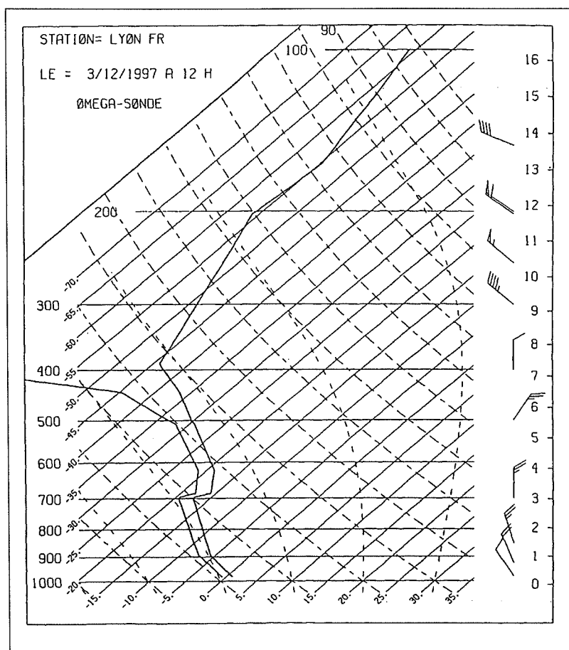
Figure III.5. : Situation météorologique générale le 3 décembre.
