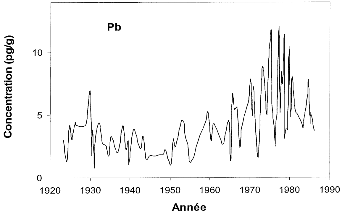
Figure 1-3 : Evolution des concentrations de Pb dans la neige de la Terre de Coats (Antarctique) entre les années 1923 et 1986 d'après Wolff et Suttie (1994).
