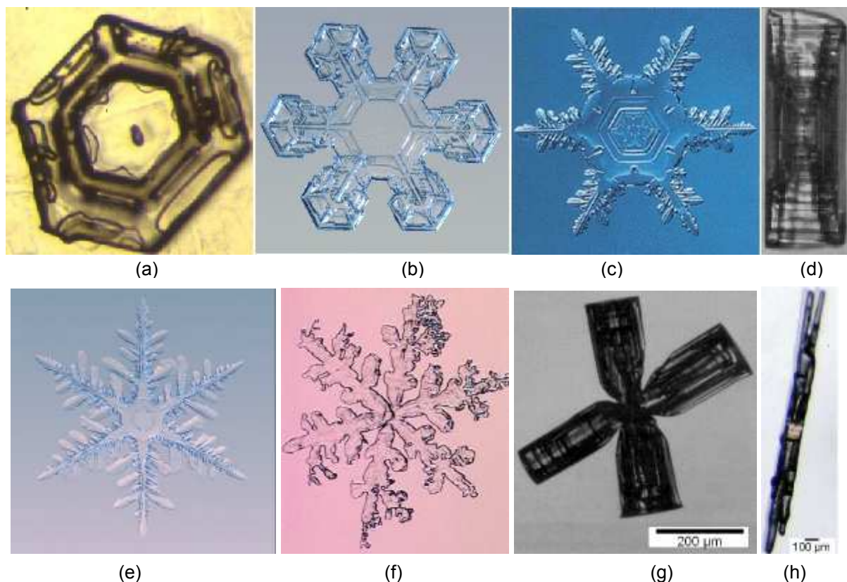
Figure II.2.1 : Observations au microscope optique de cristaux de neige prélevés lors de leur précipitation. (a) Plaquette. (b) Plaquette avec extension en étoile (Libbrecht, site web). (c) Plaquette avec extensions dendritiques (Furukawa, 1991). (d) Colonne creuse (Kobayashi et Kurado, 1987). (e) Cristal dendritique. (f) Cristal dendritique légèrement givré. (g) Cristal de 'Diamond Dust' : combinaison de 4 cristaux ayant crû à partir d'une gouttelette gelée polycristalline. (h) Aiguille.
