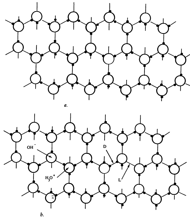
Figure II.1.5 : Structures de la glace I_h . (a) Structure parfaite. (b) Structure avec des ions H_3O^+ et OH^- , ainsi que des défauts de Bjerrum L et D.
