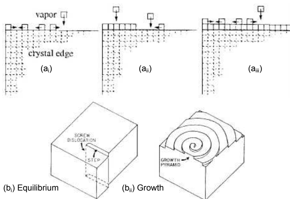
Figure II.2.7 : Mécanisme de croissance des faces cristallines (a) par nucléation homogène (d'après Nelson, 1998). Lorsqu'une marche est nucléée sur le bord d'une face les molécules s'adsorbent et la marche se propage vers le centre de la face (a i et a ii ) ; puis une nouvelle couche peut commencer à se former (a iii ).
