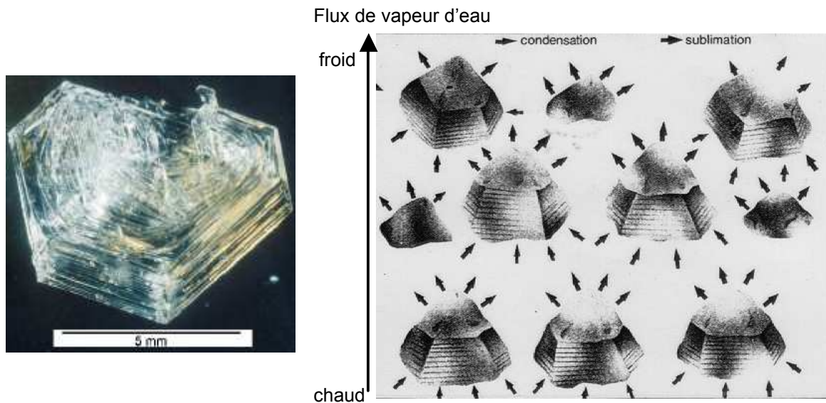
Figure II.3.7 : Mécanisme de croissance de grains anguleux sous l'effet d'un fort gradient de température ( > 15^{\circ}\text{C}/\text{m} ). Les cristaux de givre de profondeur peuvent atteindre plusieurs mm comme le montre la photographie de gauche
