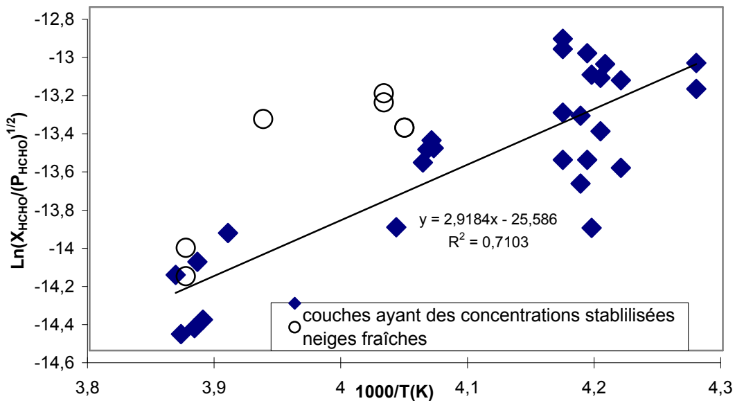
Figure III.2: Diagramme d'Arrhenius testant l'hypothèse d'une solution solide à l'équilibre thermodynamique d'après l'équation (III.2). Le calcul a été fait pour n=2 . La droite de corrélation n'inclut que les neiges dont la concentration en formaldéhyde est stable dans le temps.
