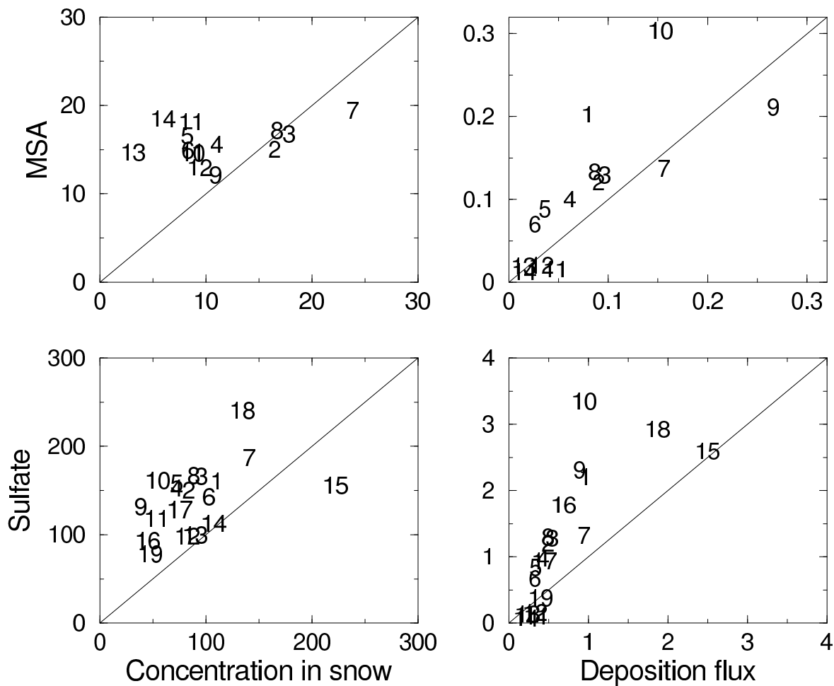
FIG. 4.13 – Comparaison des données de mesure (en abscisse) et des résultats du modèle (en ordonnée) : concentrations dans le névé et les carottes de glace (ng.g -1 , gauche) et flux de dépôt ((μmol.m -2 .d -1 ), droite) du MSA (rangée du haut) et du sulfate non marin (rangée du bas), aux sites Antarctiques de la Figure 4.11. Les données de mesure sont extraites de la compilation de Minikin et al. (1998).
