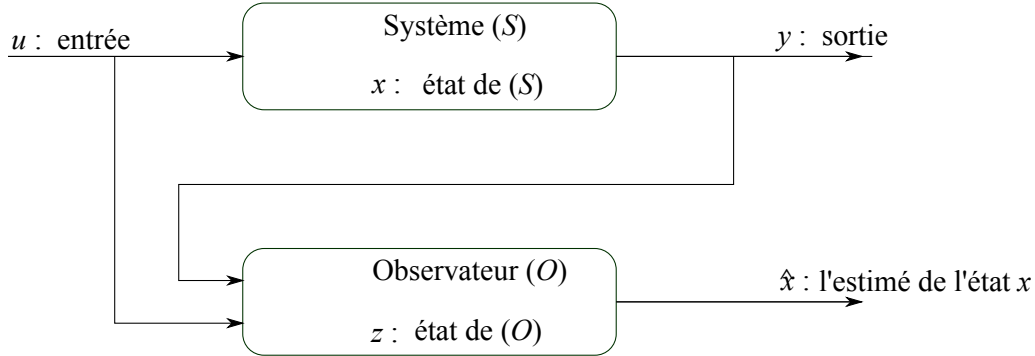
FIGURE 1.3: Observateur d'état
