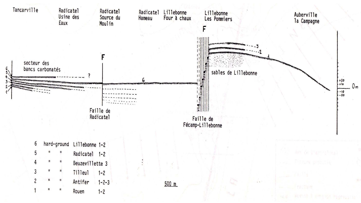
Figure II- 36 : Coupe transversale de la faille Fécamp-Lillebonne (Ragot, 1988)
