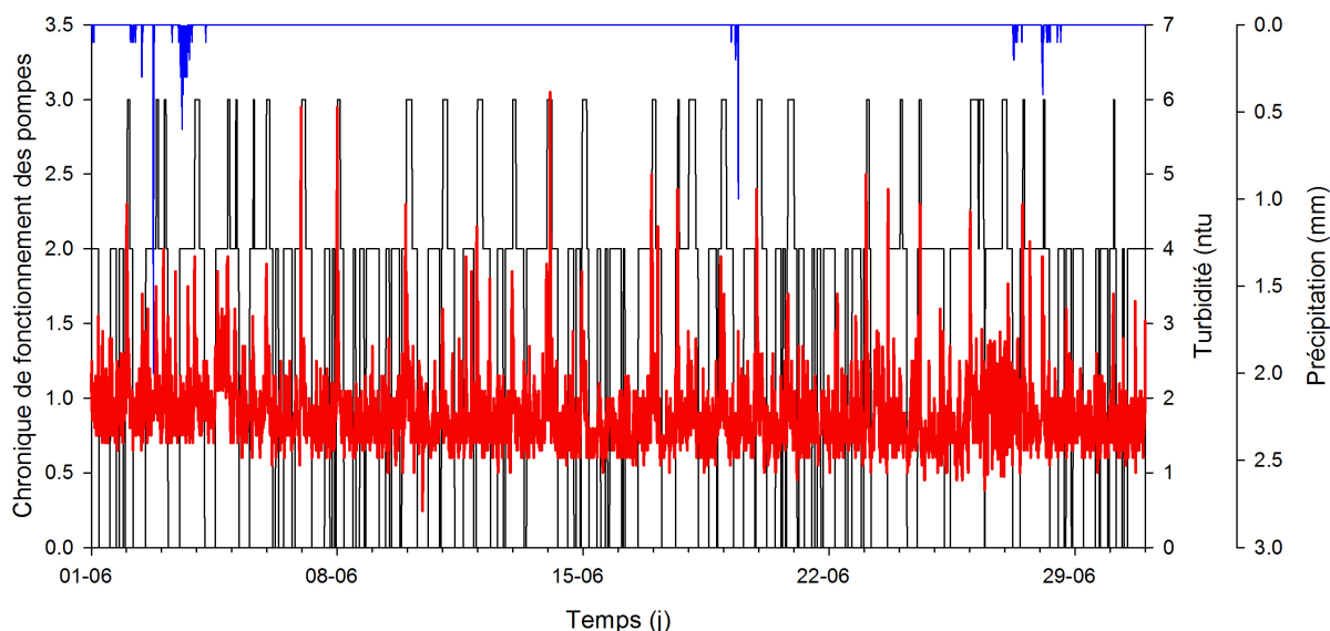
Figure IV- 2 : Mise en évidence de l'impact de la mise en route des pompes sur la turbidité de la source de la Bruisseresse
