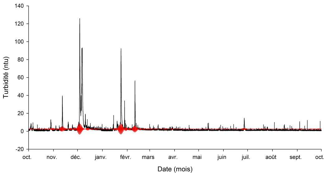
Figure III- 29 : Reconstruction du signal turbide engendré par le pompage pour la source de la Bruisseresse durant le cycle hydrologique 2008-09.
