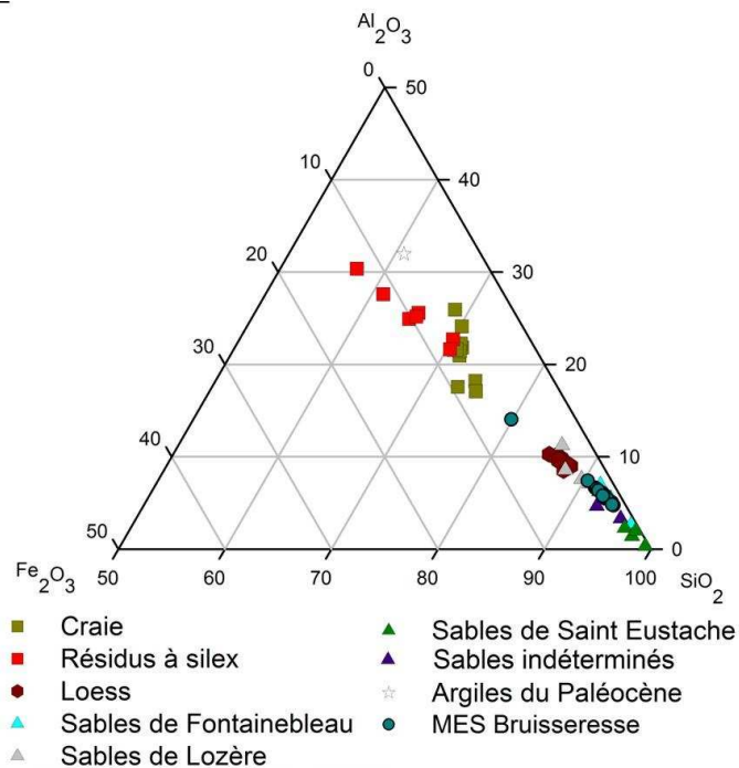
Figure IV- 5 : Comparaison de la géochimie des formations superficielles susceptibles d'être à l'origine des remplissages karstiques et des MES de la Bruisseresse
