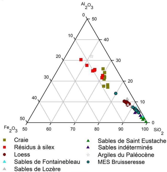
Figure II- 27 : Comparaison de la géochimie des formations superficielles susceptibles d'être à l'origine des remplissages karstiques et des MES de la Brissarthe
