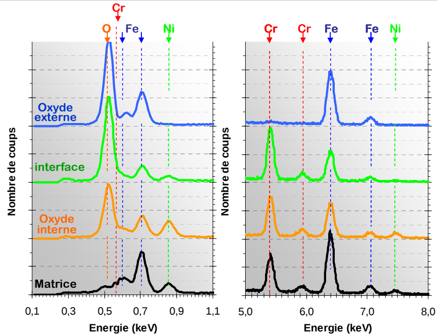
Figure IV-9 : Spectres d'émission X de l'oxyde externe, de l'interface entre les deux couches d'oxyde, de l'oxyde interne et de la matrice obtenus par EDS sur une coupe transverse d'un échantillon plan poli-miroir d'alliage 316L exposé 335 h en eau supercritique (600 °C – 250 bar)
