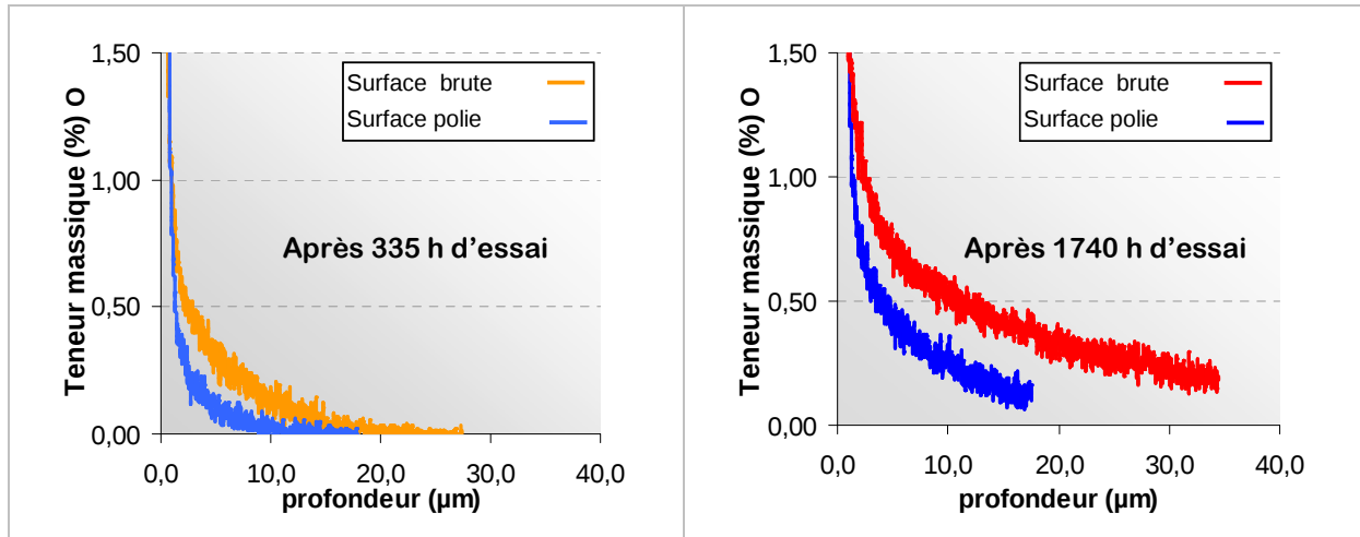
Figure III-33 : Comparaison des profils quantitatifs d'oxygène obtenus en SDL des échantillons d'alliage 690 en eau supercritique (600°C – 250 bar)
