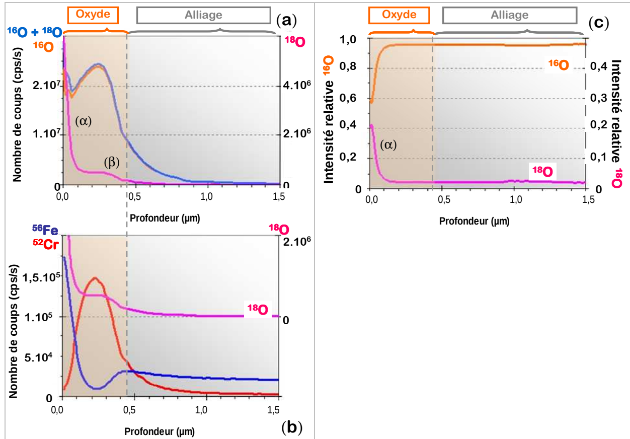
Figure IV-24 : Résultats obtenus en SIMS sur un échantillon brut d'usinage d'alliage 316L exposé 950 h en deux séquences en eau supercritique ( 600^{\circ}\text{C} – 250 bar)
