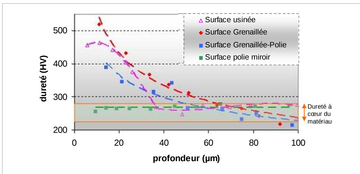
Figure II-8 : Profils de dureté des différentes surfaces étudiées dans le cas de l'alliage 316L
