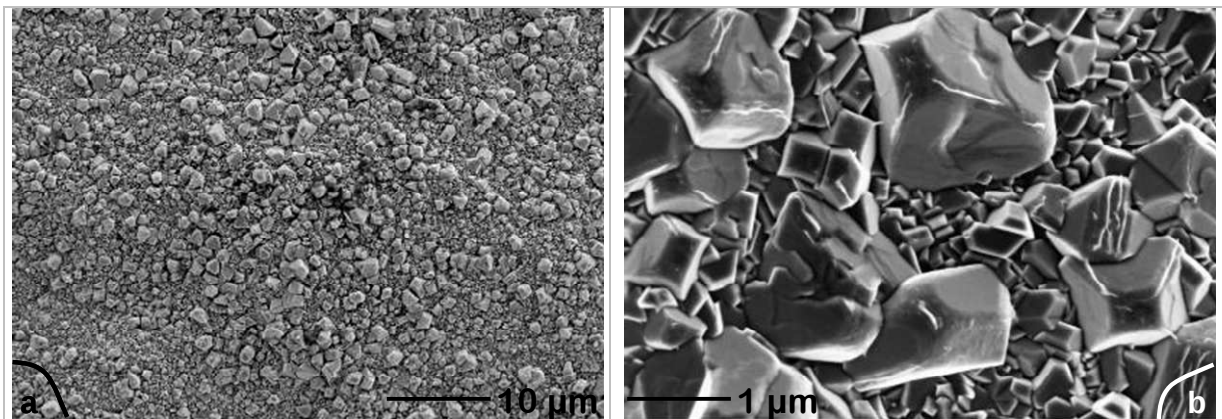
Figure IV-13 : Observations au MEB de la surface de l'oxyde formé sur un coupon plan écaillé par grenaillage d'alliage 316L exposé 1010 en eau supercritique (600°C – 250 bar) [tension d'accélération de 5 keV]
