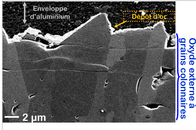
Figure IV-5 : Observations au MEB (x 2 000) en coupe transverse de l'oxyde formé sur un coupon plan poli-miroir d'alliage 316L exposé plus de 3600 h en eau supercritique (600 °C – 250 bar) [tension d'accélération de 5 keV] (voir Annexe 1).
