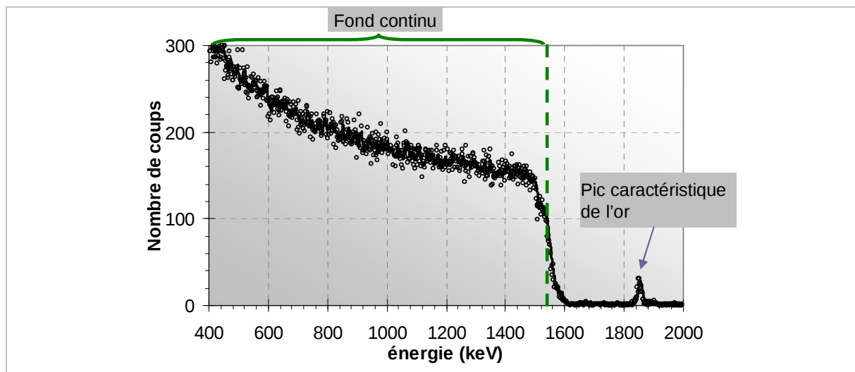
Figure III-23 : Spectre expérimental obtenu en RBS sous un faisceau incident de ^4\text{He}^+ [d'énergie d'incidence de 2 MeV] sur un coupon poli-miroir d'alliage 690 marqué à l'or (non exposé en eau supercritique)
