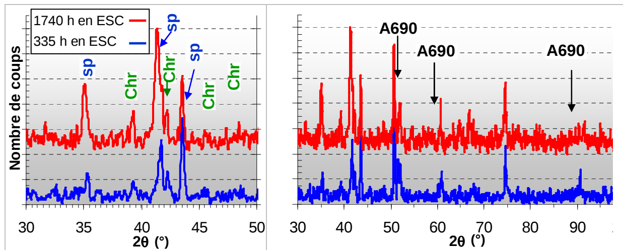
Figure III-16 : Diffractogrammes obtenus en mode rasant ( 1^\circ d'incidence) des oxydes formés sur des coupons plans polis-miroir d'alliage 690 exposé 335 h et 1740 h en eau supercritique (600 °C – 250 bar).
