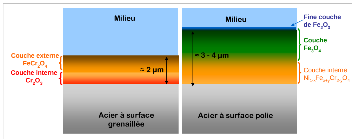
Figure I-8 : Schéma de la couche d'oxyde formée sur l'acier 800H lorsque la surface oxydée en eau supercritique est soit grenillée, soit polie (500 °C, 25 MPa) d'après Tan et al. [TAN08a].
