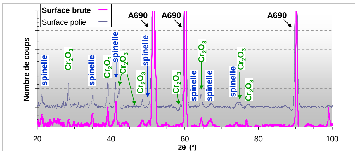
Figure III-34 : Diffractogramme en mode \theta - 2\theta de l'oxyde formé sur un coupon plan poli-miroir d'alliage 690 exposé 840 h en eau supercritique (600°C – 250 bar)
