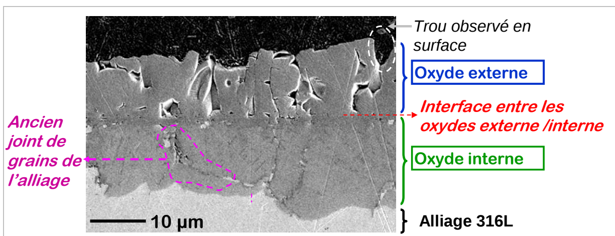
Figure IV-4 : Observations au MEB (x 2 000) en coupe transverse de l'oxyde formé sur un coupon plan poli-miroir d'alliage 316L exposé 335 h en eau supercritique (600 °C – 250 bar) [tension d'accélération de 5 keV].
