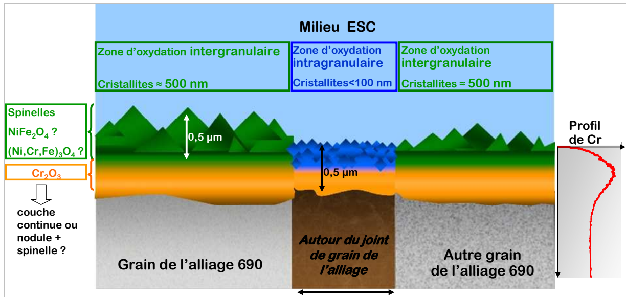
Figure III-6 : Schéma récapitulatif de la couche d'oxyde formée sur un échantillon plan poli-miroir d'alliage 690 exposé 840 h en eau supercritique (600 °C – 250 bar)
