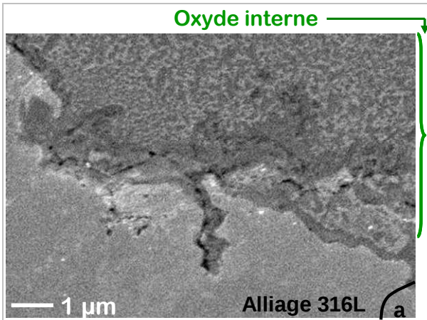
Figure IV-6 : Observations au MEB en coupe transverse de l'oxyde formé sur des coupons plans polis-miroir d'alliage 316L et d'alliage 304L exposés en eau supercritique (600 °C – 250 bar) [tension d'accélération de 5 keV]
