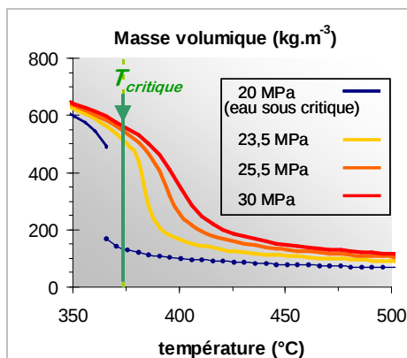
Figure I-2 : Masse volumique de l'eau en fonction de la température et de la pression
