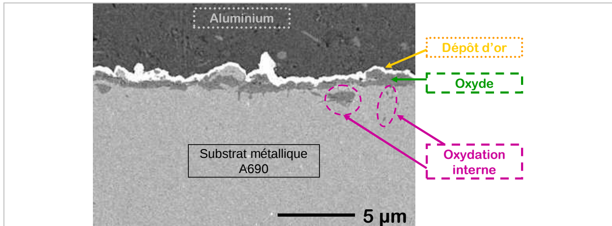
Figure III-3 : Observation au MEB en électrons rétrodiffusés ( \times 5\,000 ) d'une coupe transverse d'un échantillon (tête de capsule) plan poli-miroir exposé 840 h en eau supercritique (600 °C – 250 bar) [tension d'accélération de 5 keV]
