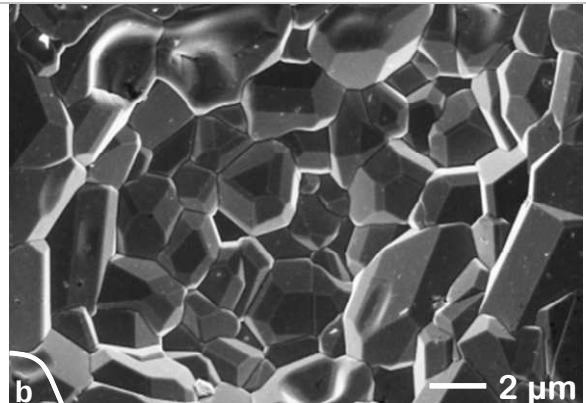
Figure IV-3 : Observations au MEB (x 5 000) de la surface de la couche d'oxyde formée sur un coupon plan poli-miroir d'alliage 316L exposé 335 h en eau supercritique (600 °C – 250 bar) [tension d'accélération de 5 keV]
