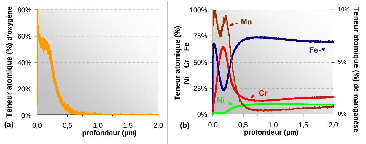
Figure IV-18 : Profils obtenus en SDL sur un échantillon brut d'usinage d'alliage 316L exposé 335 h en eau supercritique (600 °C – 250 bar)
