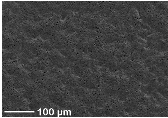
Figure IV-2 : Observation au MEB (x 200) de la surface de la couche d'oxyde formée sur un coupon plan poli-miroir d'alliage 316L exposé 335 h en eau supercritique (600 °C – 250 bar) [tension d'accélération de 5 keV] montrant un relief bosselé.
