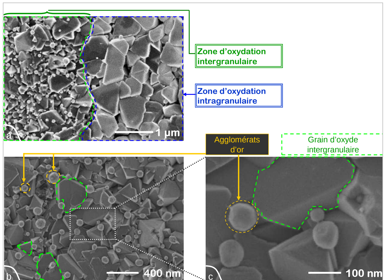
Figure III-22 : Observation au MEB en électrons secondaires de l'oxyde formé sur un coupon plan poli-miroir d'alliage 690 marqué à l'or exposé 335 h en eau supercritique (600°C – 250 bar)
