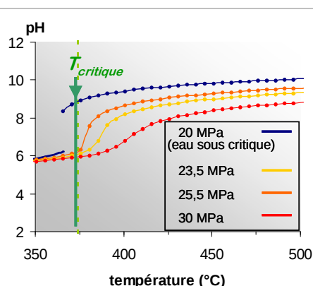
Figure I-5 : pH de l'eau en fonction de la température et de la pression.
