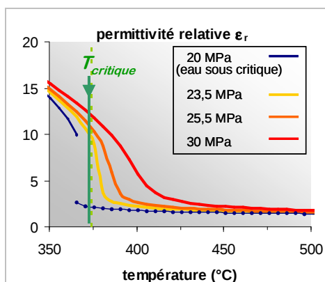
Figure I-4 : Permittivité relative de l'eau en fonction de la température et de la pression
