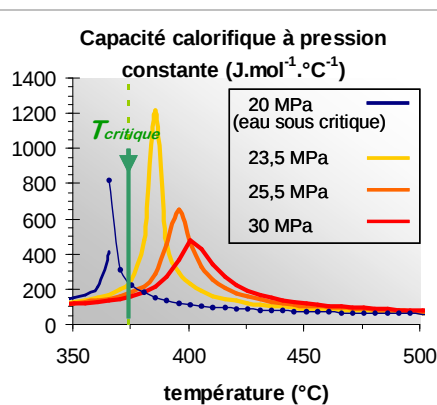
Figure I-3 : Capacité calorifique à pression constante de l'eau en fonction de la température et de la pression
