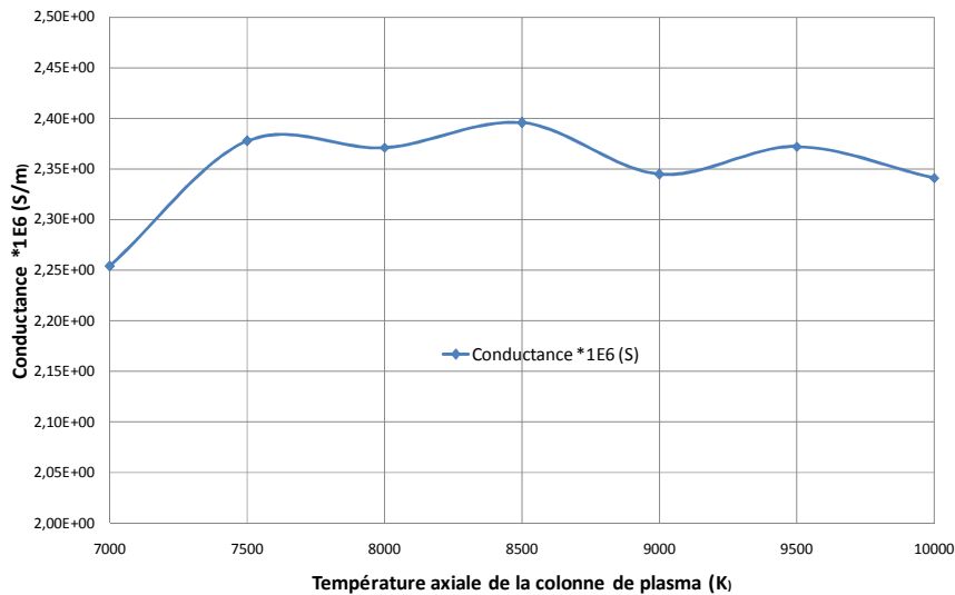
Figure 3.14 : Conductance calculée de la colonne de plasma en fonction de la température axiale.
