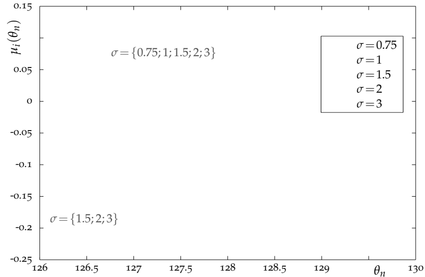
FIGURE 3.2: Représentations graphiques des moyennes \mu_0, \mu_1 et de leurs approximations, en négligeant la quantification, \widehat{\mu}_0, \widehat{\mu}_1 en fonction de \theta_n \in [126;130] et pour \sigma_n = \{0.75; 1; 1.5; 2; 3\} . Dans un souci de clarté, les valeurs sont multipliées par \sigma_n^2 afin que \widehat{\mu}_0 = -1/8 .
