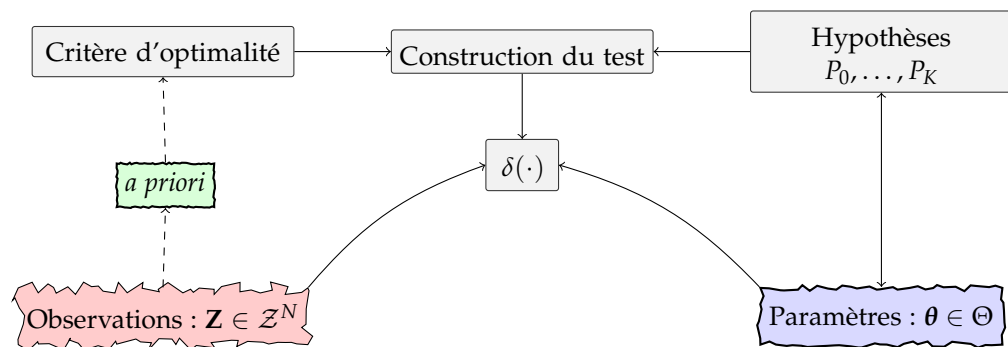
FIGURE 2.10: Illustration d'un test statistique d'hypothèses.
