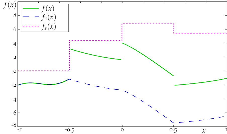
FIGURE 5.3: Illustration du théorème 5.1 sur la décomposition d'une fonction f continue par morceaux en une somme d'une fonction f_c continue et d'une fonction f_s constante par morceaux.
