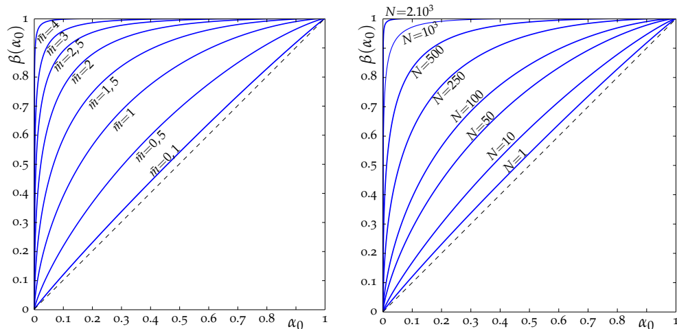
(a) Courbes COR du test le plus puissant à partir d'un seul échantillon \bar{m} = \{0.1; 0.5; 1; 1.5; 2; 2.5; 3; 4\} (b) Courbes COR du test le plus puissant à partir de N = \{1; 10; 50; 100; 250; 500; 1000; 2000\} et \bar{m} = 0.1
