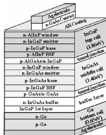
Figure II-27 : Schéma d'une cellule triple-jonctions. La cellule top a un grand gap pour absorber les photons dans le bleu. La cellule middle a un gap dans le proche infrarouge, et la cellule bottom a un petit gap dans l'infrarouge pour capter les photons de petite énergie. Les cellules sont connectées entre elles par les jonctions tunnel. La couche tampon entre Ge et InGaAs sert à adapter leur paramètre de maille (195) .
