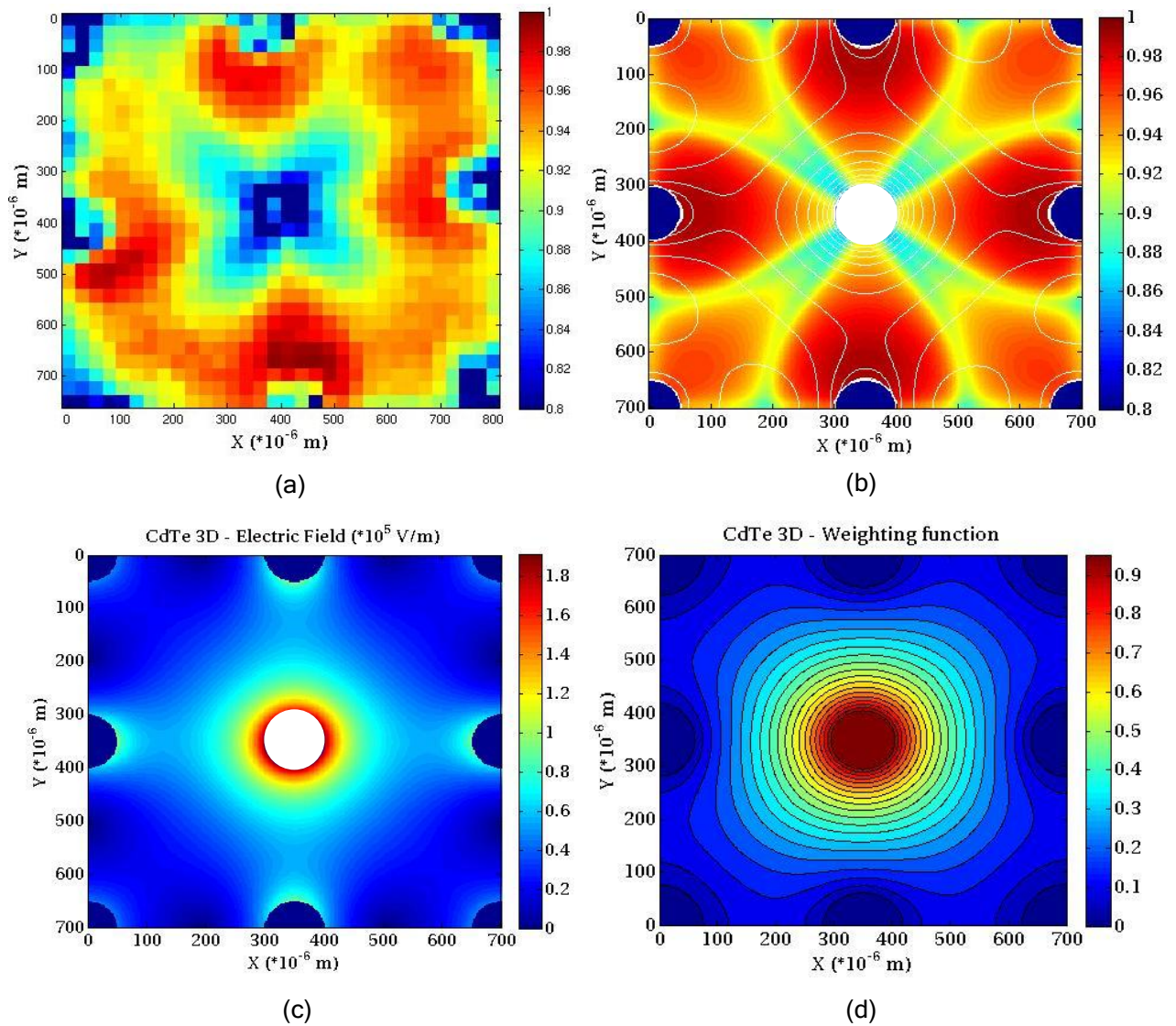
Figure V-14 : (a) Cartographie du canal du pic à 60 keV normalisé et (b) Cartographie de la CIE simulée et lignes isopotentielle pour le détecteur 3D à base de CdTe:Cl (échelle de couleur entre 0,8 (bleu foncé) et 1 (rouge foncé)) et distributions (c) du champ électrique et (d) de la fonction de pondération calculées par simulation, les disques bleus correspondent aux cathodes et le disque blanc à l'anode sur les cartographies simulées
