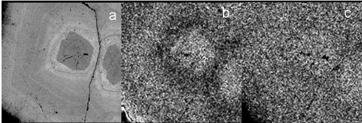
Figure 57 : Images de la surface polie de l'échantillon kazakh en MEB BSE (a) et cartographie élémentaire microsonde associée de Ca (b) et Mo (c).
