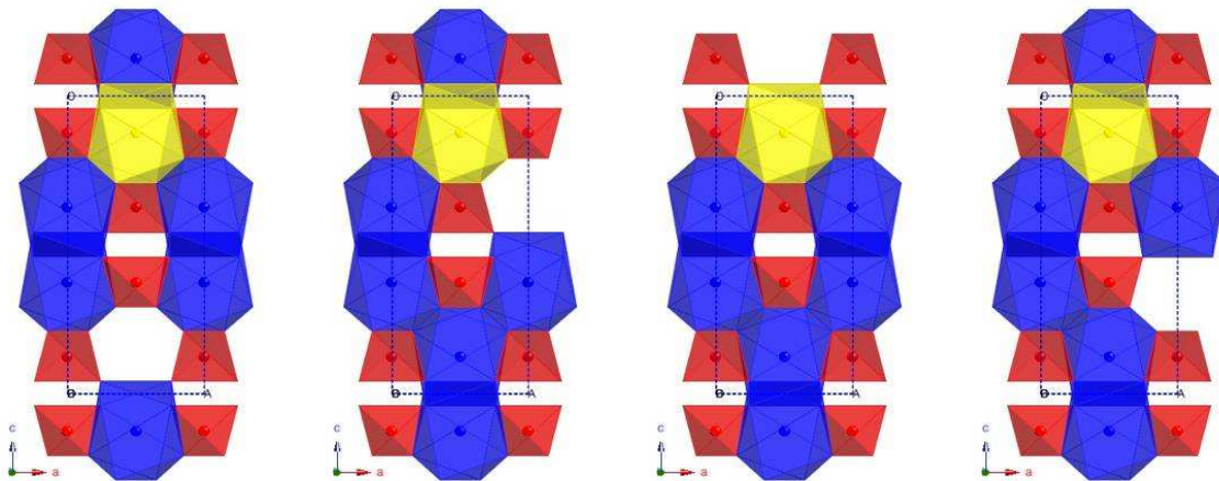
Figure 84 : Quatre possibilités de compensation par une lacune de l'ajout d'une terre rare dans la structure cristalline. Les polyèdres de coordination du calcium sont représentés en bleu, du molybdène en rouge et de l'euprium en jaune.
