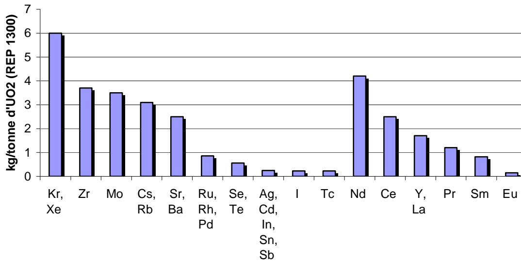
Figure 3 : Masses produites de produits de fission par un réacteur REP 1300 CEA par tonne de combustible \text{UO}_2 utilisé [4].
