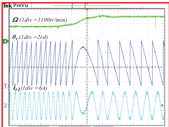
(a) Transition du mode hypo au mode hyper synchrone (b) Transition du mode hyper au mode hypo synchrone Fig.III. 49 : Résultats expérimentaux durant le changement de mode de fonctionnement.
