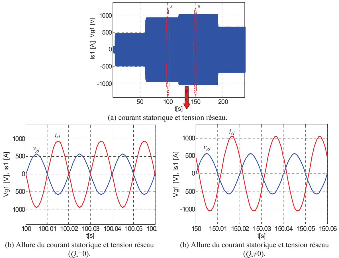
Fig. II. 44 : Evolution du courant statorique et rotorique de la MADA.
