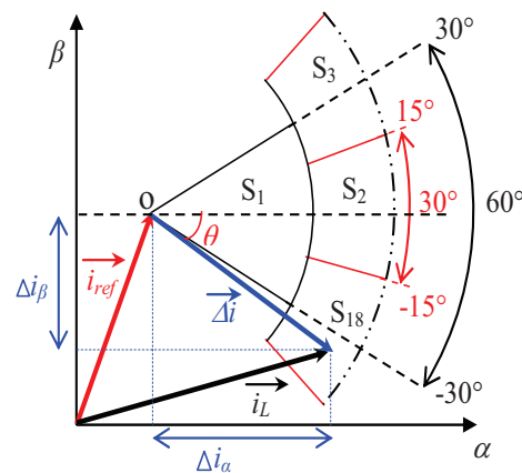
Fig.III. 34 : Angle entre deux secteurs consécutifs
