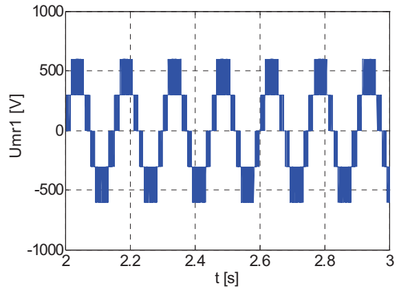
(f) Tension à la sortie du convertisseur coté rotor.
