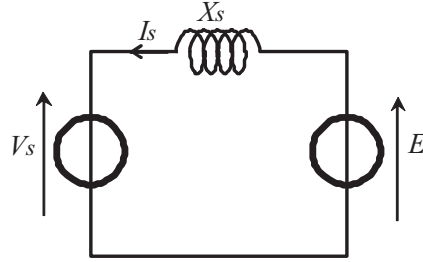
Fig. IV. 18 : Schéma équivalent simplifié par phase de la MADA.
