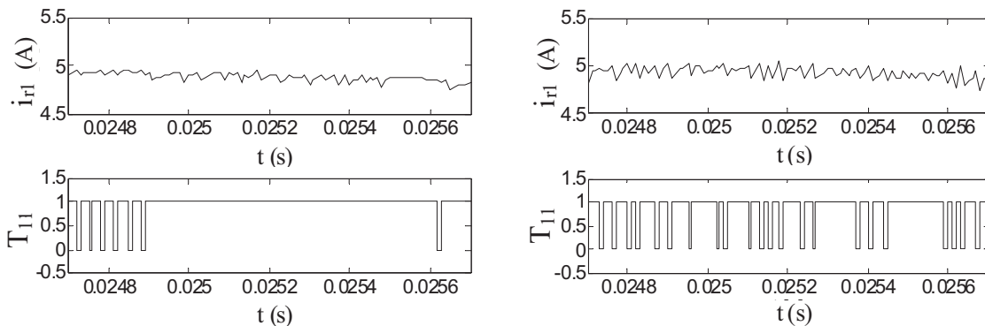
(a) Avec l'hystérésis conventionnel à trois niveaux.
