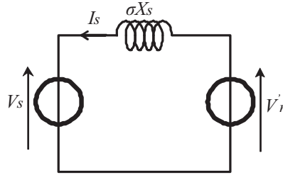
Fig. IV. 24 : Schéma équivalent simplifié par phase de la MADA.
