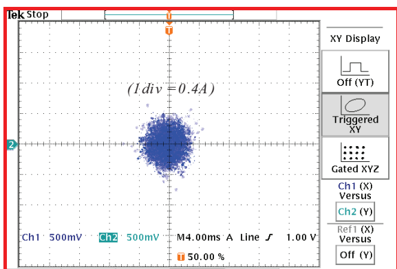
(c) Erreur du courant rotorique dans le plan \alpha\beta
