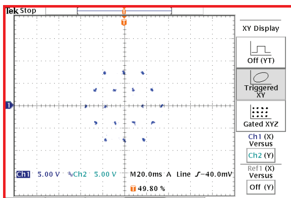
(d) Les 27 vecteurs de tension appliqués
