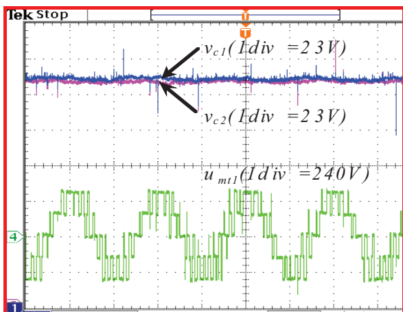
(a) ch1 : Tensions aux bornes des deux condensateurs, ch2 : Tension composée à la sortie du convertisseur.
