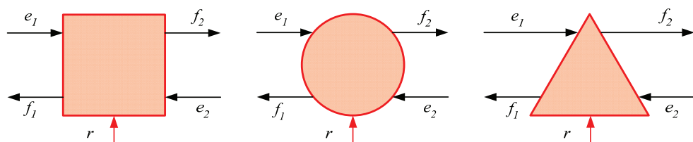
Fig. A.4 : REM des éléments de conversion pour un gyrateur.
