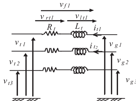
Fig. II. 21 : Filtre coté réseau.
