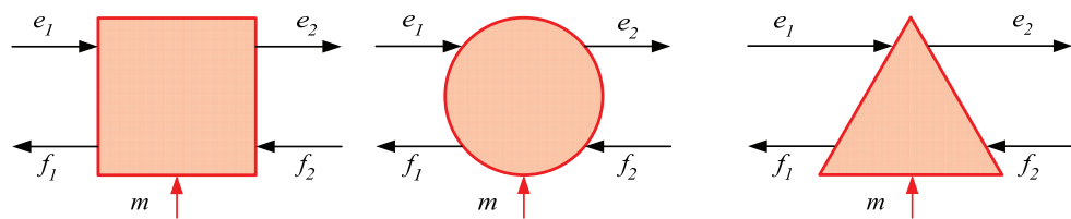
Fig. A.3 : REM d'un élément d'accumulation.
