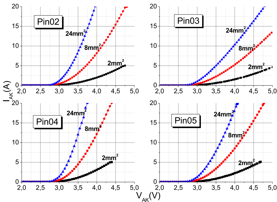
FIGURE 3.33: Exemple de caractéristiques en direct des diodes 2, 8 et 24 mm^2 pour les 4 wafers à 25^{\circ}C pour des impulsions de courant égales à 256 \mu s .
