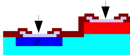
FIGURE 4.21: Vue en coupe de ouverture 2 .
