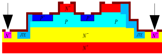
FIGURE 4.18: Vue en coupe de ouverture 1
