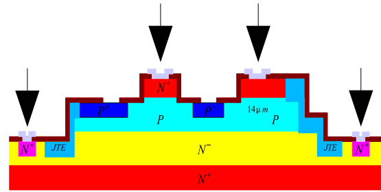
FIGURE 4.19: Vue en coupe de métal 1 .
