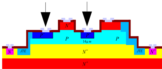
FIGURE 4.20: Vue en coupe de métal 2
