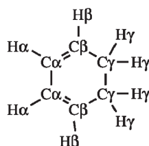
1,3-cyclohexadiene (CYD)
