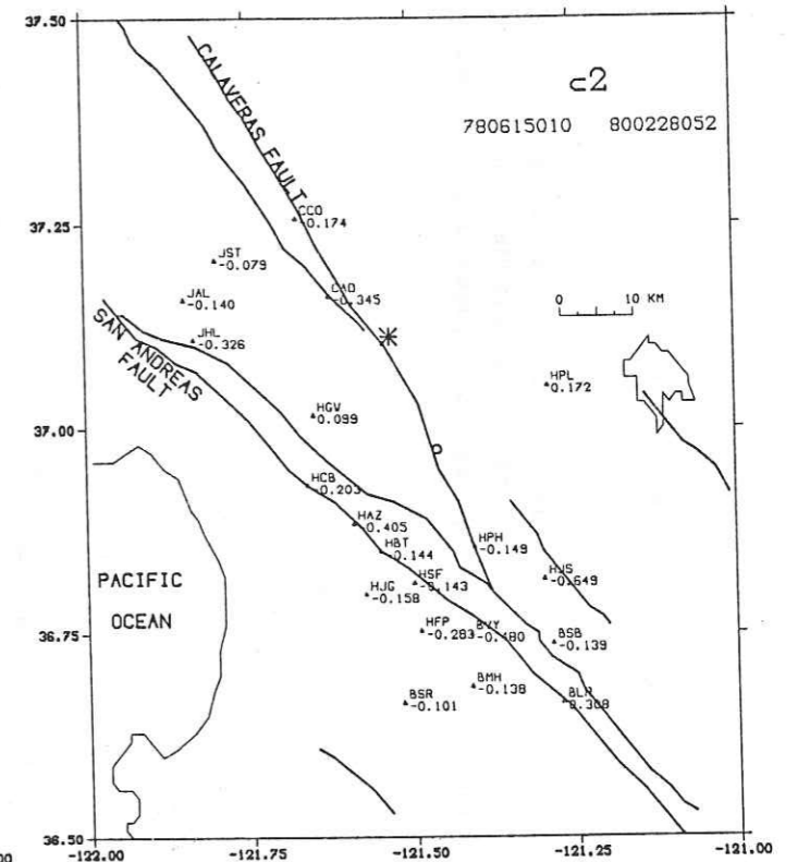
Figure 8 (Suite). Carte des valeurs de M_{IG} , moyenne pondérée du logarithme du rapport spectral: doublets A723, A867, S7, C2.
