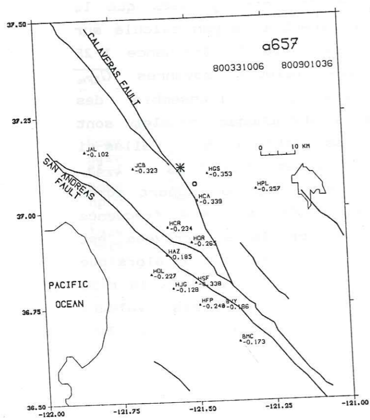
Figure 8. Carte des valeurs de M_{IG} , moyenne pondérée du logarithme du rapport spectral: doublets A712, A713, A657, S4.
