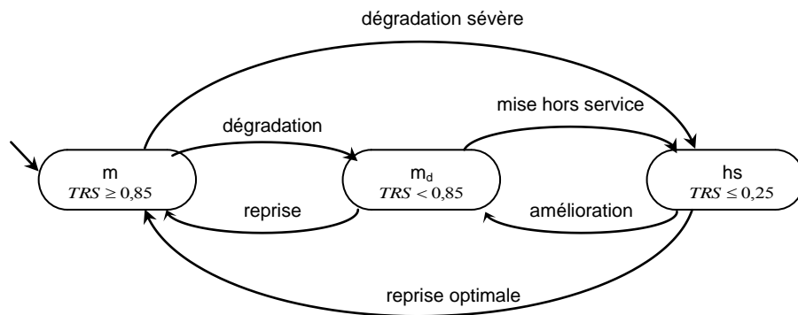
Figure 5.2: Le modèle automate du TRS d'un composant réparable
