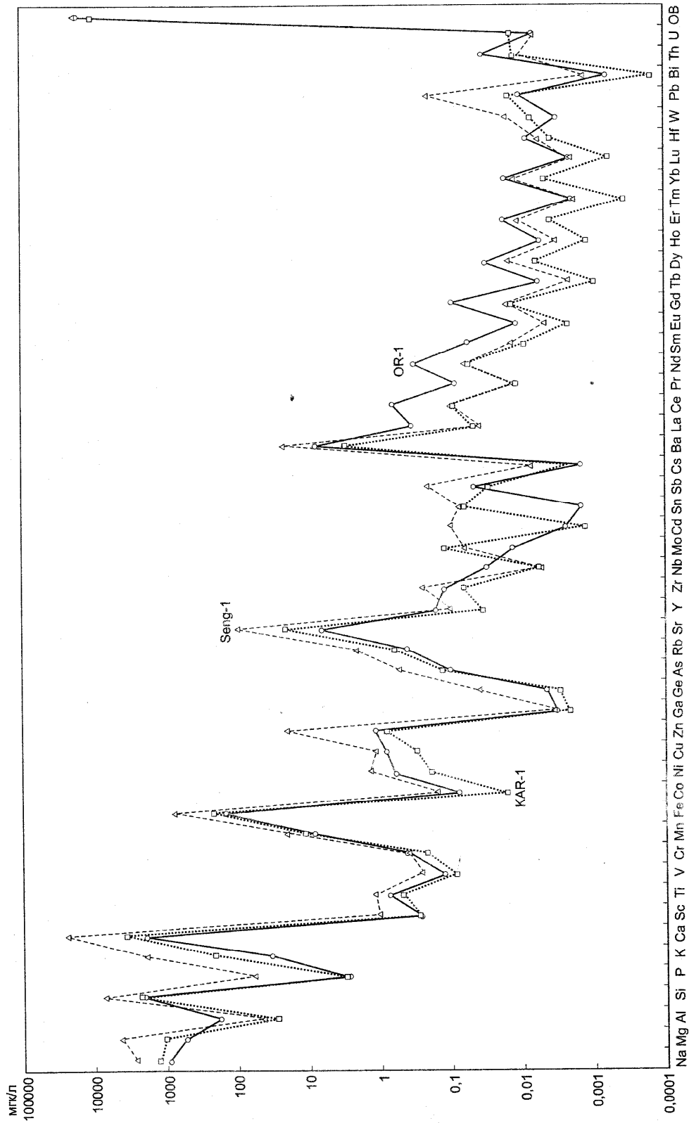
Рис. 1. Сравнение содержания элементов в (фильтрах 0.2 мкм речного стока двух регионов: KAR-1 — р. Палеёвки; OR-1 — р. Восточный (борисальская зона) и Seng-1 — р. Сеньга (Мещерская низменность)
