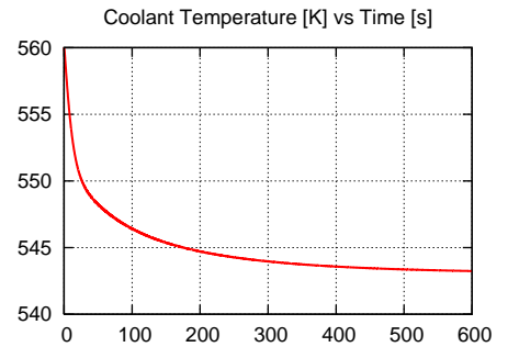
FIG. 5.5 – Jeu initial des paramètres thermiques ou cinétiques (a) et résultats (b) calculés par CheckPoint pour le transitoire "UTOP min" du CANDU ^{nat}U (BOC) avec \Delta\rho_{min} = -390 pcm.
