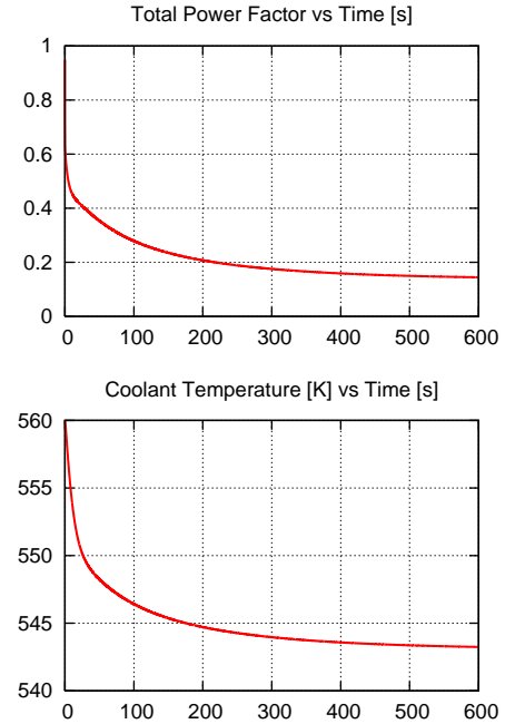
FIG. 5.5 – Jeu initial des paramètres thermiques ou cinétiques (a) et résultats (b) calculés par CheckPoint pour le transitoire "UTOP min" du CANDU ^{nat}U (BOC) avec \Delta\rho_{min} = -390 pcm.
