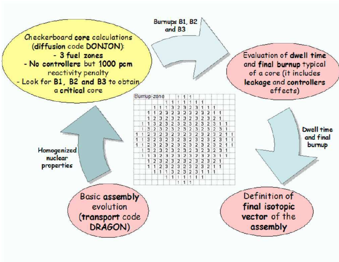
FIG. 2.8 – Schéma de calcul “cœur-équivalent” adapté au REP, basé sur la méthode “time-average” à 3 zones de burnup.
