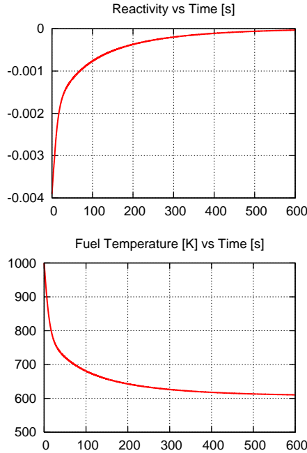
FIG. 5.5 – Jeu initial des paramètres thermiques ou cinétiques (a) et résultats (b) calculés par CheckPoint pour le transitoire "UTOP min" du CANDU ^{nat}U (BOC) avec \Delta\rho_{min} = -390 pcm.
