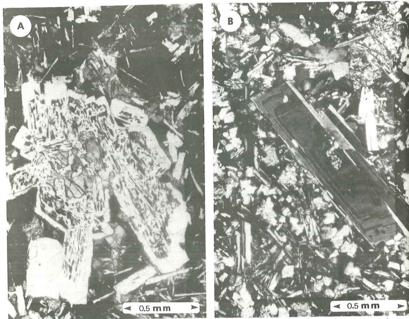
FIG 80 - Plagioclase zoné dans une microdolerite
