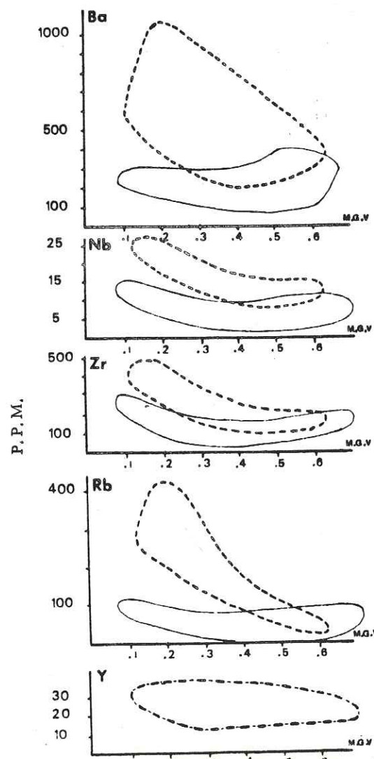
FIG 21 - Mise en évidence des deux lignées (même légende que la fig. ).
