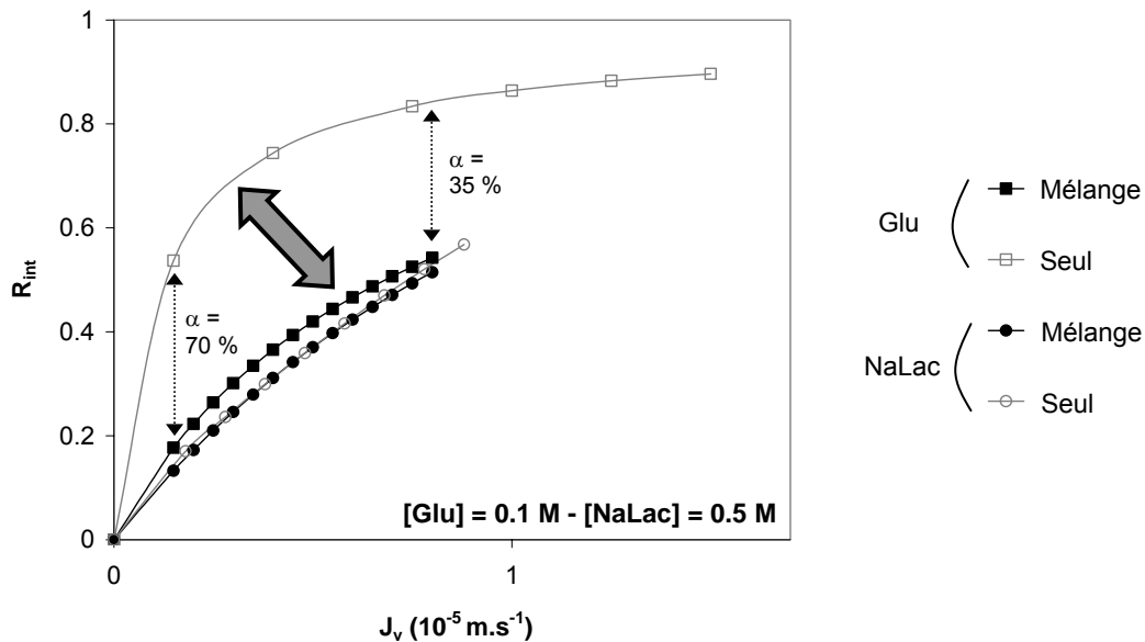
Figure IV-6 . Mélanges glucose / lactate de sodium - Rétention intrinsèque - Comparaison avec les rétentions des solutés seuls en solution - Membrane DK15 - [Glu] = 0.1 M - [NaLac] = 0.5 M
