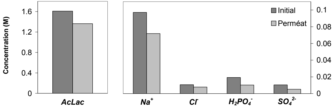
Figure V-5 . Jus n°3 - Composition initiale et après filtration - \Delta P = 20 bar
