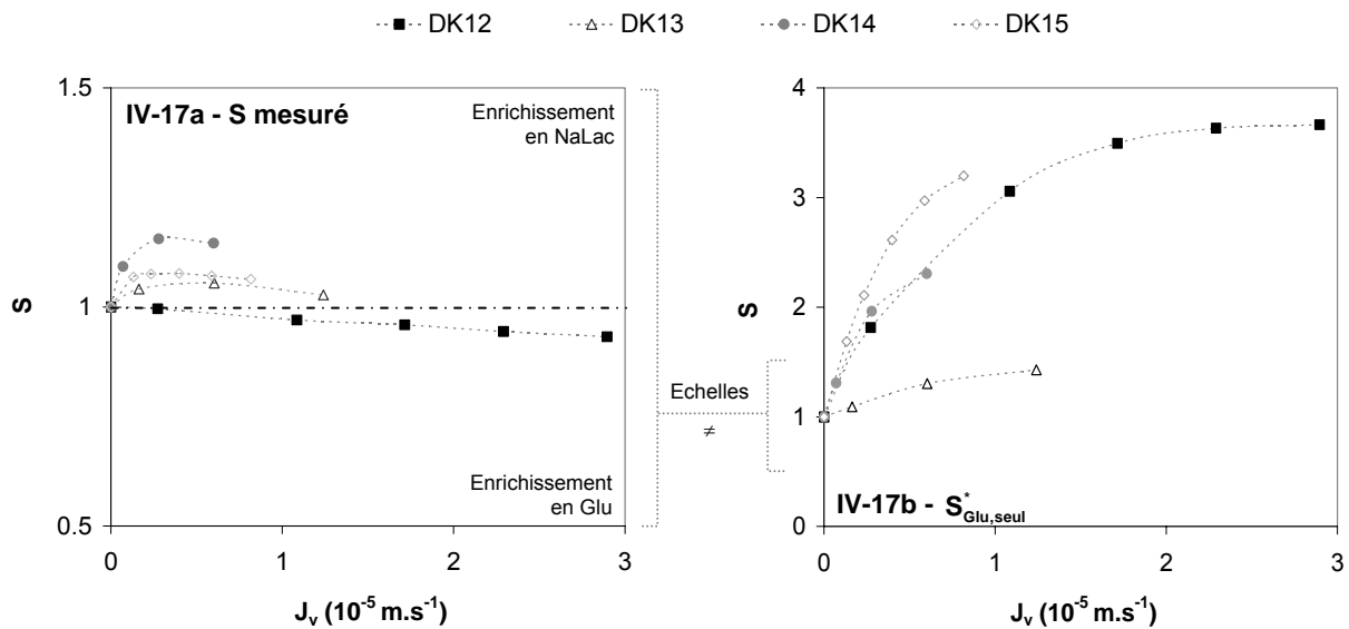
Figure IV-17 . Mélange glucose / lactate de sodium - Evolution du facteur de séparation S en fonction de J_v - [Glu] = 0.1 \text{ M} - [NaLac] = 0.5 \text{ M} - Membranes DK12, DK13, DK14, DK15
