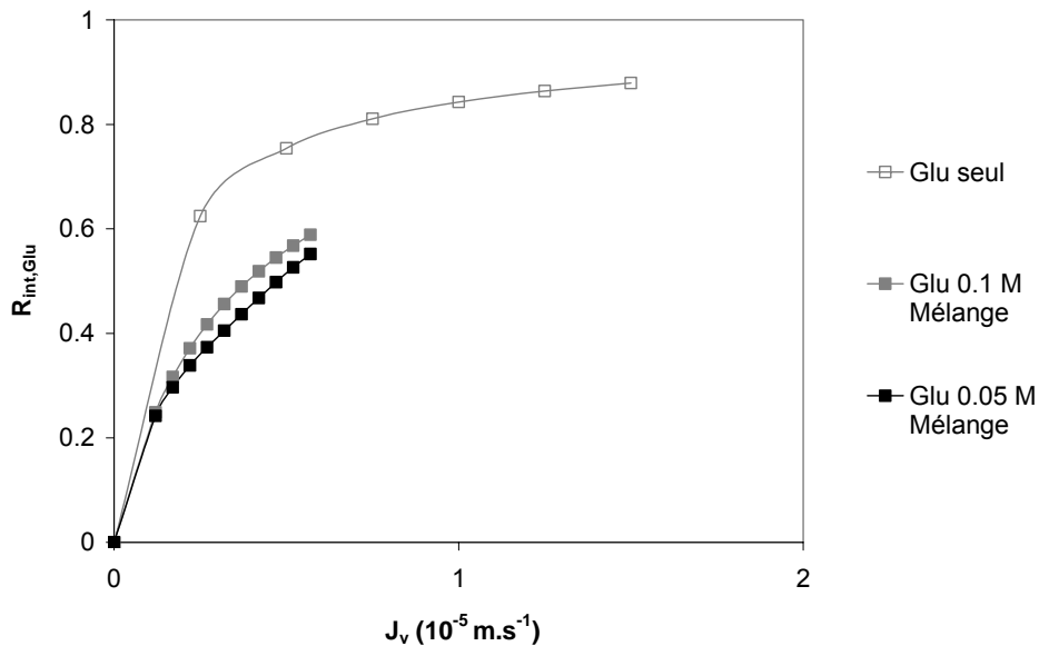
Figure IV-9 . Mélange glucose / lactate de sodium - Rétention intrinsèque du glucose - Influence de la concentration initiale en glucose - Membranes DK14 - [NaLac] = 0.5 M
