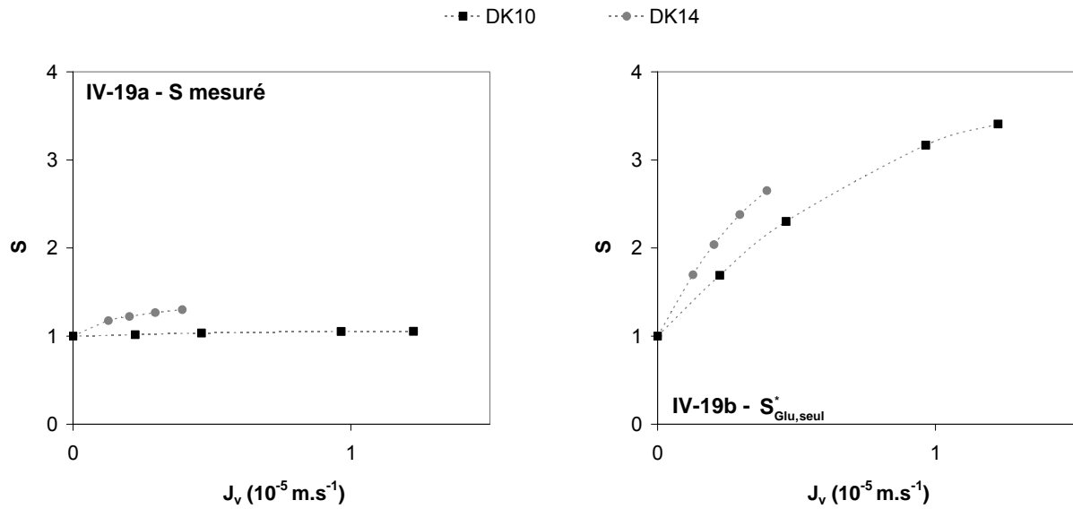
Figure IV-19 . Mélange glucose / lactate de sodium - Evolution du facteur de séparation S en fonction de J_v - [Glu] = 0.1 M - [NaLac] = 1 M - Membranes DK10 et DK14
