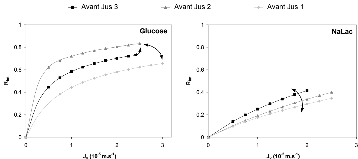
Figure V-2 . Caractéristiques de la membrane (DK17) - Rétentions intrinsèques de glucose et NaLac avant chaque filtration - [Glu] = 0.1 \text{ M} - [NaLac] = 0.5 \text{ M}
