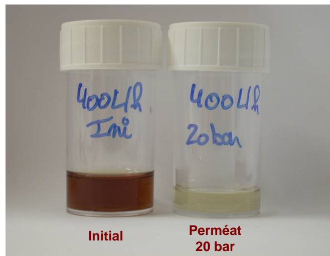
Fig. V-12 . Décoloration opérée par la nanofiltration d'un jus de fermentation brut clarifié - Jus n°3 - \Delta P = 20 bar
