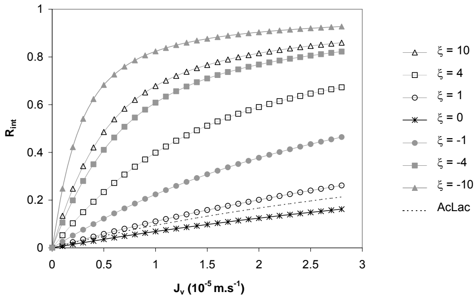
Figure II-18 . Rétention intrinsèque d'une solution de lactate de sodium en fonction du flux volumique de perméation J_v . Modèle "DSPM" - r_p = 0.5 \text{ nm} et L/\varepsilon = 1.5 \text{ }\mu\text{m} . Influence du rapport \xi = X_d/c_m .
